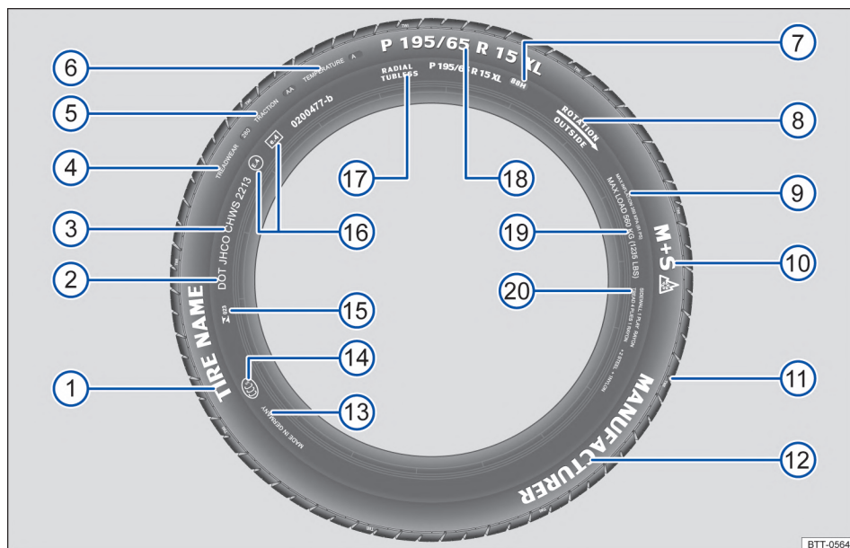
Fig. 194 Inscripción de los neumáticos internacional (ejemplo).
