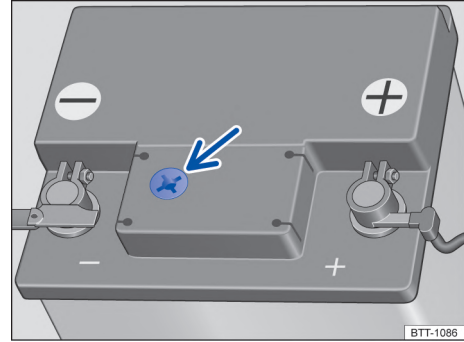
Fig. 187 En el compartimento del motor: ejemplo de posición del visor en el lado superior de la batería del vehículo.
