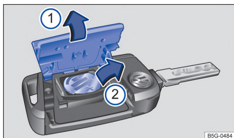
Fig. 52 Llave del vehículo: sustituir la pila.
