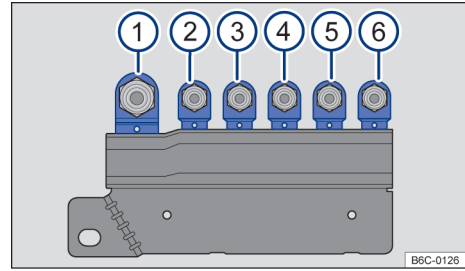
Fig. 173 En el compartimento del motor encima de la batería: disposición de los fusibles.
