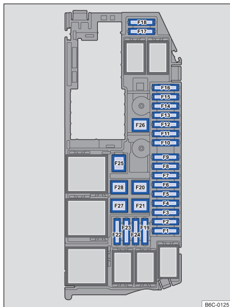
Fig. 172 En el compartimiento del motor: disposición de los fusibles.
