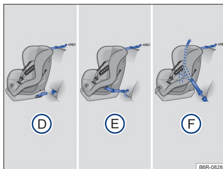
Fig. 42 En el asiento trasero: las figuras D y E muestran el principio de fijación del sistema de retención infantil en los ojales de retención inferiores y con el cinturón de fijación superior. La figura F muestra la fijación del sistema de retención para niños con el cinturón de seguridad del vehículo y con el cinturón de fijación superior.
