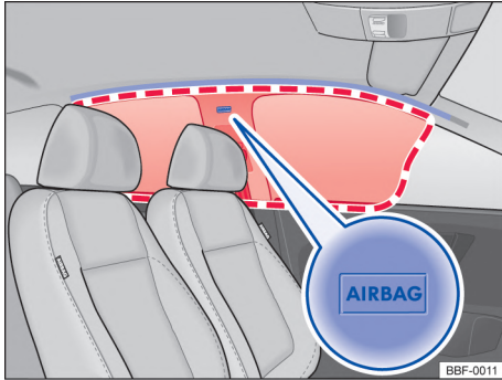
Fig. 40 En el lado izquierdo del vehículo: ubicación de montaje y área de expansión del airbag para cabeza.
