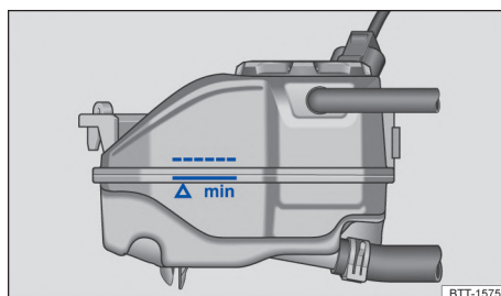
Fig. 184 En el compartimento del motor: marca en el depósito de expansión del líquido refrigerante del motor.
