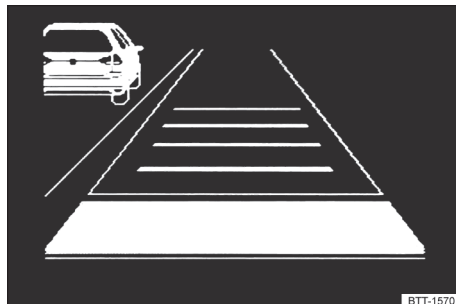
Fig. 98 En la pantalla del cuadro de instrumentos: vehículo más lento detectado en el carril izquierdo (representación esquemática).
