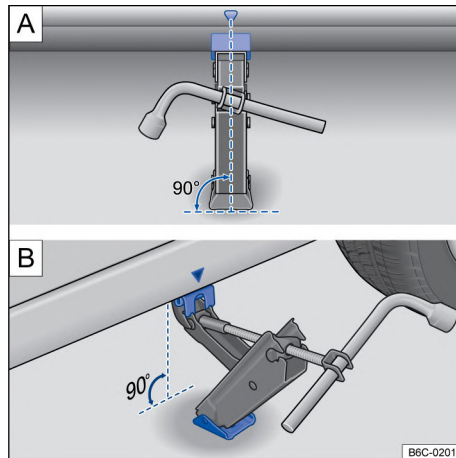
Fig. 200 Puntos de apoyo del gato y gato posicionado atrás en el lado izquierdo trasero del vehículo.
