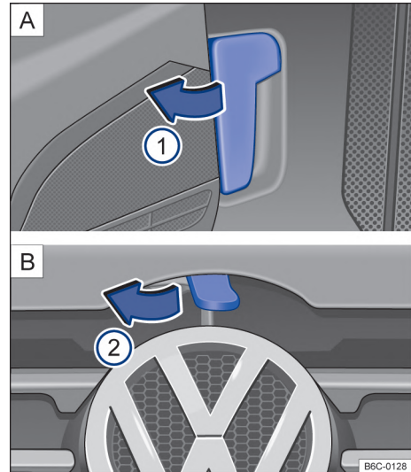
Fig. 178 A Palanca de desbloqueo de la tapa del compartimento del motor en la zona reposapiés del conductor. B Palanca de desbloqueo en la parte inferior de la tapa del compartimento del motor.
