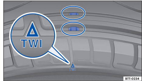
Fig. 192 Perfil del neumático: indicadores de desgaste.
