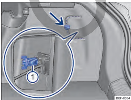
Fig. 206 En el maletero: desmontar la cubierta y retirar el tornillo mariposa ① (fragmento ampliado).
