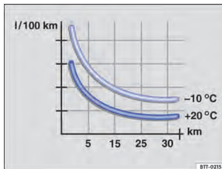
Fig. 92 Consumo de combustible en l/100 km en 2 temperaturas ambiente diferentes.
