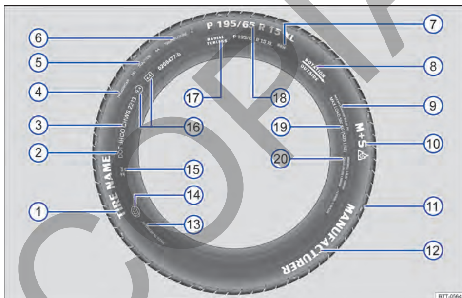
Fig. 185 Inscripción de los neumáticos internacional (ejemplo).
