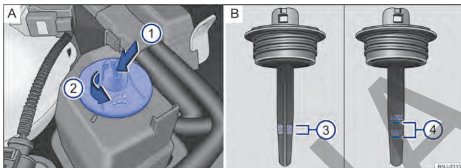
Fig. 86 En el vano del motor (variante 1): A Tanque del fluido de la dirección hidráulica. B Marcas para controlar el nivel del líquido de la dirección asistida.
