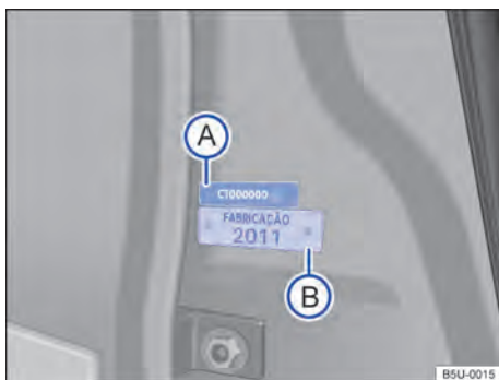
Fig. 196 En la columna de la puerta delantera derecha: etiqueta con el número de bastidor parcial (A) y placa del modelo, año de fabricación (B) .
