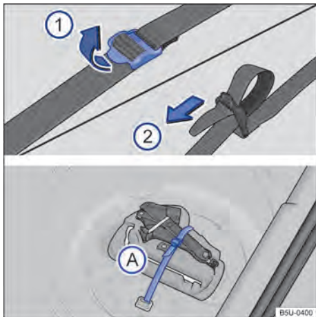
Fig. 148 En el maletero: cinta de fijación de la caja de herramientas y caja de herramientas de a bordo.
