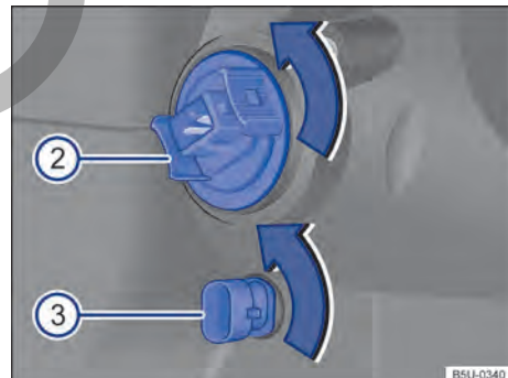
Fig. 153 En el compartimento del motor: vista trasera del farol delantero 2 indicadores de dirección y 3 luz de posición.
