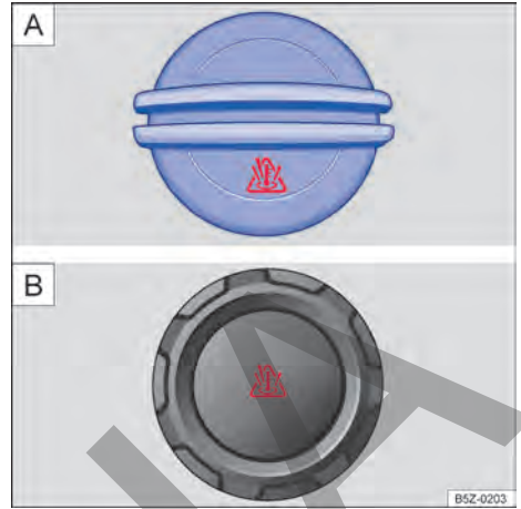
Fig. 176 En el compartimento del motor: A) tapa del depósito de expansión del líquido de refrigeración del motor (variante 1) o B) tapa del depósito de expansión del líquido de refrigeración del motor (variante 2).
