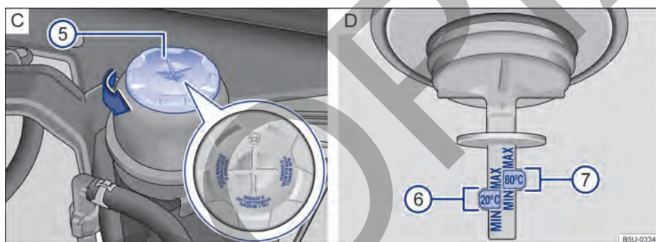
Fig. 87 En el vano del motor (variante 2): C Tanque del fluido de la dirección hidráulica. D Marcas para controlar el nivel del líquido de la dirección asistida.
