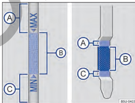
Fig. 173 Varilla de medición del aceite con marca de nivel de aceite del motor. ▶
