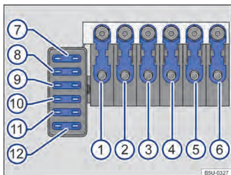
Fig. 165 Caja de fusibles.
