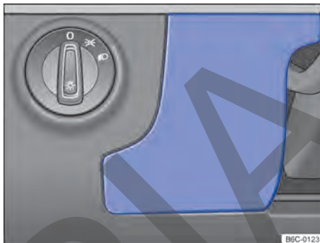
Fig. 171 Del lado del conductor en el panel de instrumentos: cubierta de la caja de fusibles.
