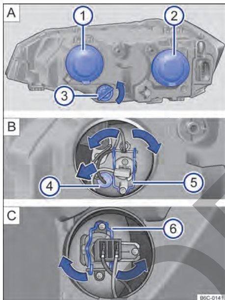
Fig. 163 En el compartimento del motor: ① faro alto y luz de posición, ② faro bajo y ③ intermitente.
