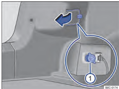
Fig. 165 En el maletero: desmontar la cubierta y retirar el tornillo mariposa ① (fragmento ampliado).
