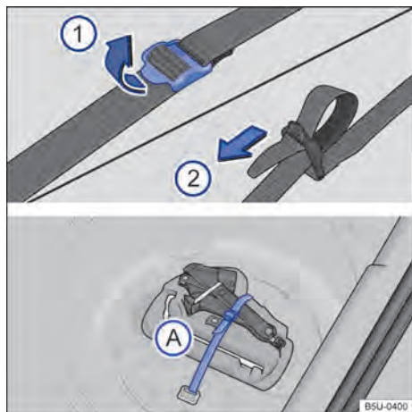
Fig. 156 En el maletero: cinta de fijación de la caja de herramientas y caja de herramientas de a bordo.
