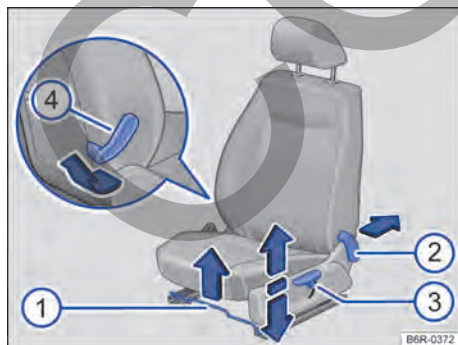
Fig. 63 En el asiento delantero: comandos.
