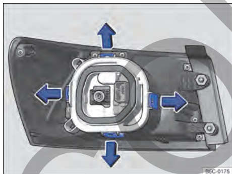
Fig. 166 Linterna trasera: desmontar el portalámparas.
