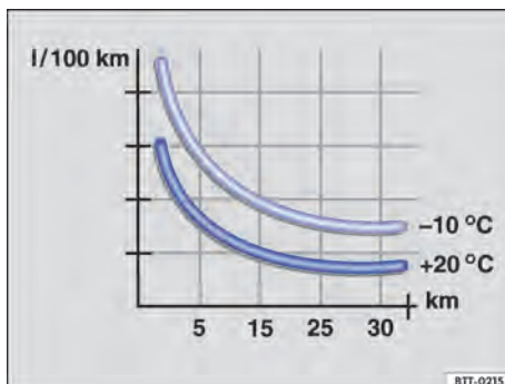
Fig. 85 Consumo de combustible en l/100 km en 2 temperaturas ambiente diferentes.
