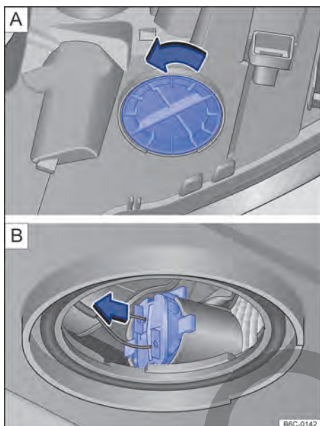
Fig. 162 Farol delantero, por debajo: cubierta del indicador de dirección.
