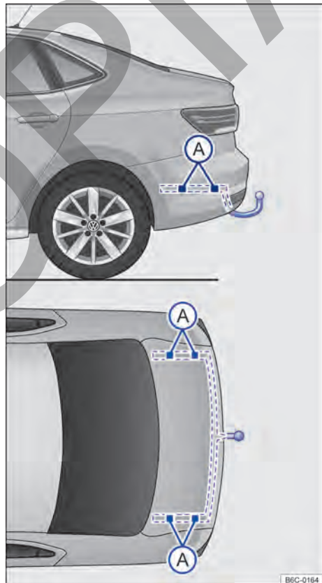
Fig. 153 Puntos de fijación para el montaje posterior de un enganche para remolque. ▶
