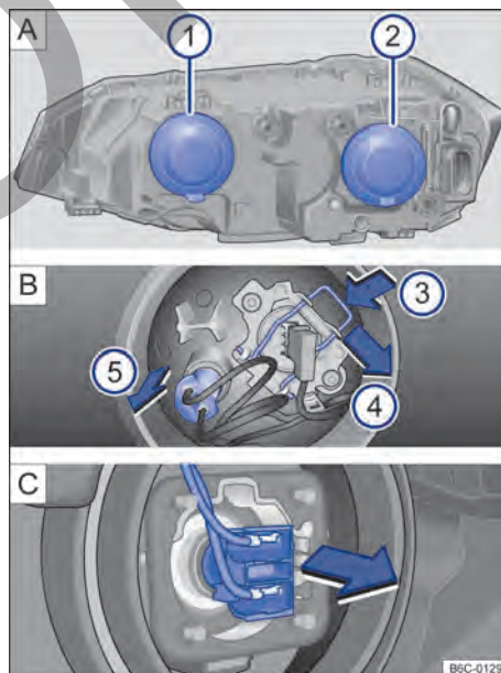
Fig. 161 En el compartimiento del motor: ① faro alto y luz de posición y ② faro bajo. ▶
