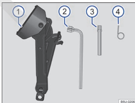
Fig. 143 Componentes de las herramientas de a bordo.
