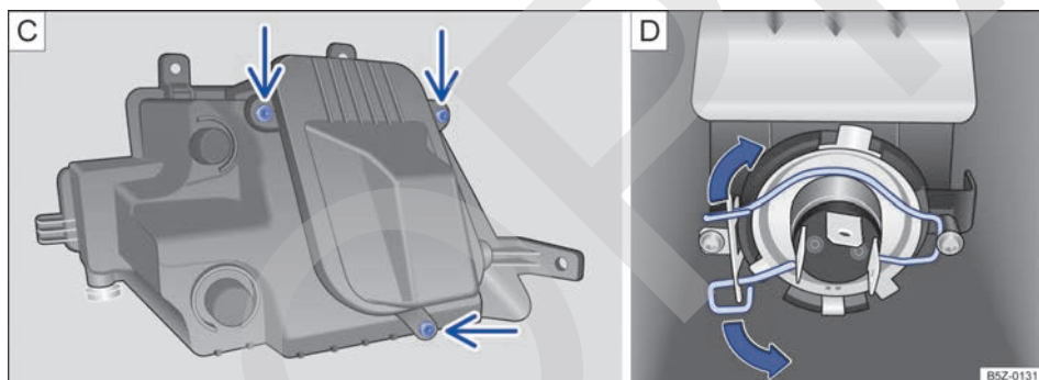
Fig. 151 En el paragolpes delantero: C retirar los tornillos de la cubierta de la bombilla y D bombilla del farol de neblina.
