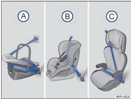
Fig. 19 Las ilustraciones (A), (B) y (C) muestran la fijación del sistema de retención infantil sólo con el cinturón de seguridad del vehículo.
