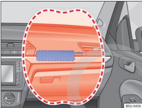
Fig. 17 Ubicación y radio de expansión del airbag frontal del acompañante.
