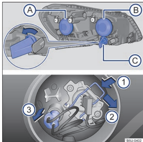
Fig. 147 En el compartimento del motor: vista trasera del farol delantero con cubierta de goma (lado izquierdo de la ilustración) - (A) farol bajo (B) farol alto y luz de posición y (C) indicador de dirección. Vista trasera del farol delantero sin la cubierta de goma (lado derecho de la ilustración): ① resorte de bloqueo de la bombilla del farol y ② luz de posición.
