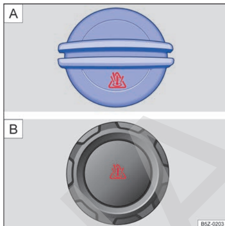
Fig. 172 En el compartimento del motor: A tapa del depósito de expansión del líquido refrigerante del motor (variante 1) o B tapa del depósito de expansión del líquido refrigerante del motor (variante 2).
