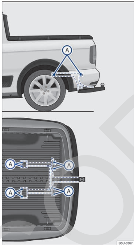
Fig. 137 Puntos de fijación para el montaje posterior de un enganche para remolque.
