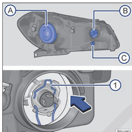
Fig. 145 En el compartimento del motor: vista trasera del farol delantero con cubierta de goma (lado izquierdo de la ilustración): A farol bajo / alto B indicadores de dirección y C luz de posición. Vista trasera del farol delantero sin la cubierta de goma (lado derecho de la ilustración): 1 resorte de bloqueo de la bombilla del farol bajo / alto.
