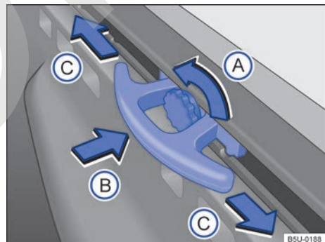
Fig. 132 En el compartimento de carga: soporte deslizante para vehículos con capota marítima.
