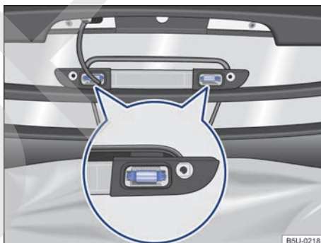
Fig. 157 Linterna de freno elevada: remover la lámpara incandescente de iluminación del compartimento de carga.
