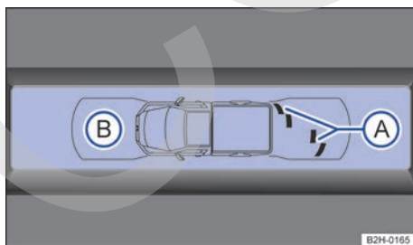
Fig. 105 Indicación del display del control de distancia de aparcamiento (display monocromático): (A) obstáculo reconocido en el segmento. (B) zona registrada delante del vehículo.
