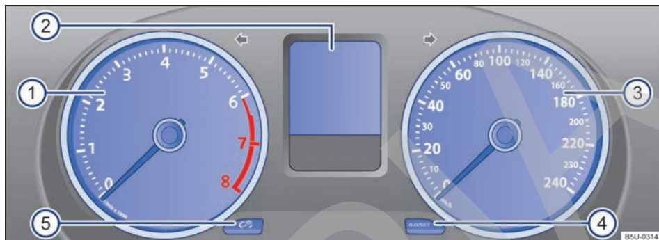
Fig. 34 Panel de instrumentos en el panel de instrumentos (variante 1).
