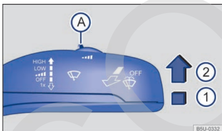
Fig. 79 Palanca de los limpiaparabrisas: ajustar la sensibilidad del sensor de lluvia (A).
