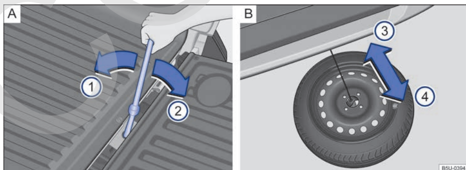
Fig. 180 A En el compartimento de carga: acceso a la rueda de emergencia. B Debajo del vehículo: rueda de emergencia totalmente en el piso y extracción de debajo del vehículo.
