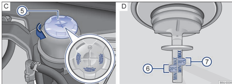
Fig. 99 En el compartimento del motor (variante 2): C Depósito del líquido de la dirección asistida. D Marcas para controlar el nivel del líquido de la dirección asistida.
