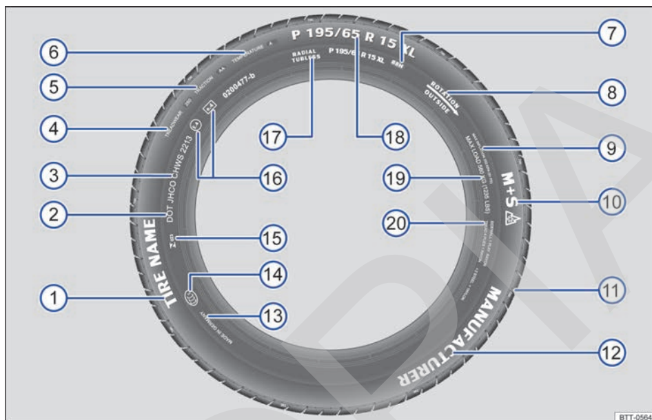
Fig. 182 Inscripción de los neumáticos internacional (ejemplo).
