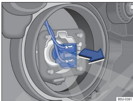
Fig. 148 Acceso a la bombilla del farol bajo.
