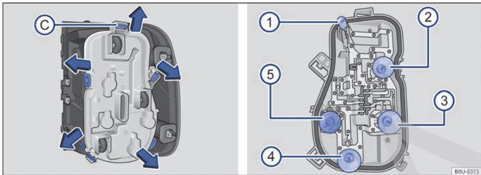
Fig. 153 Linterna trasera: C desmontar el portalámparas y 1 , 2 , 3 , 4 y 5 desmontar las bombillas.
