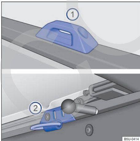
Fig. 130 En el compartimento de carga: soportes fijos ① para vehículos sin capota marítima y ② para vehículos con capota marítima.
