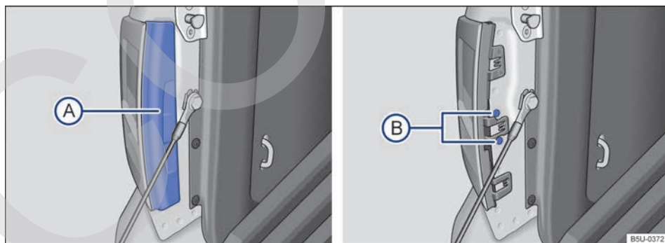
Fig. 152 En el compartimento de carga: desinstalar la cubierta, retirar los tornillos de fijación. ▶
