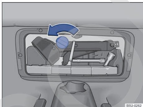
Fig. 142 Palanca de fijación de caja de herramientas de a bordo.
