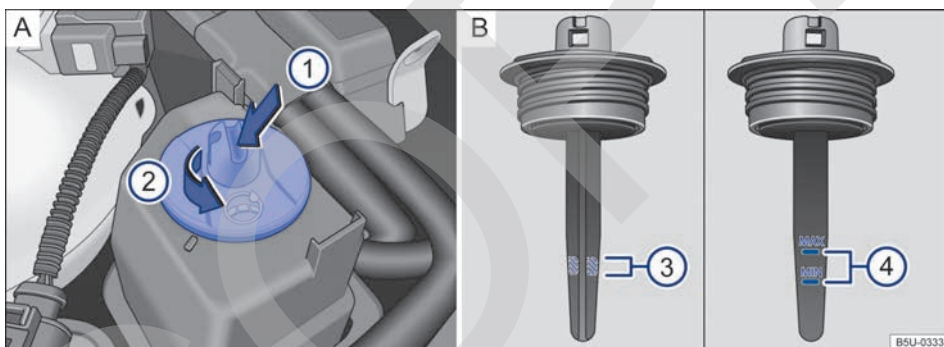
Fig. 98 En el compartimento del motor (variante 1): A Depósito del líquido de la dirección asistida. B Marcas para controlar el nivel del líquido de la dirección asistida.
