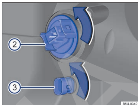
Fig. 146 En el compartimento del motor: vista trasera del farol delantero 2 indicadores de dirección y 3 luz de posición.
