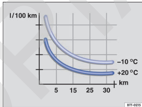
Fig. 94 Consumo de combustible en l/100 km en 2 temperaturas ambiente distintas.
