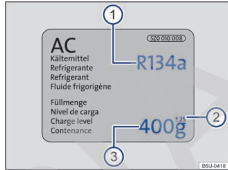
Fig. 194 Información del aire acondicionado.
