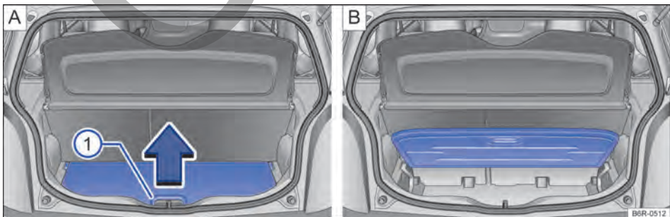
Fig. 93 A: piso variable del maletero rebatido hacia arriba. B: piso variable del maletero abierto.
