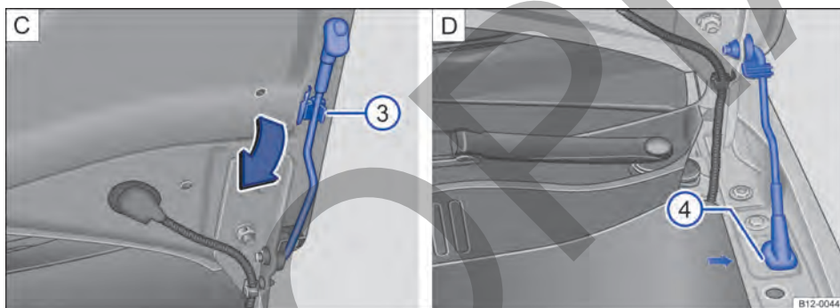
Fig. 153 C: varilla de sujeción de la tapa del compartimento del motor. D: tapa del motor protegida con la varilla de sujeción de la tapa.
