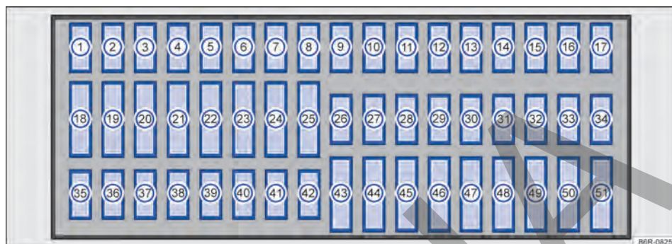
Fig. 145 Caja de fusibles.
