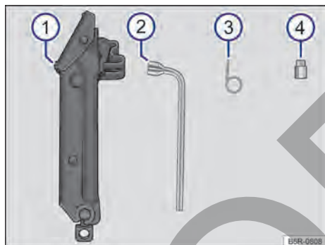
Fig. 132 Representación esquemática: componentes de las herramientas de a bordo.
