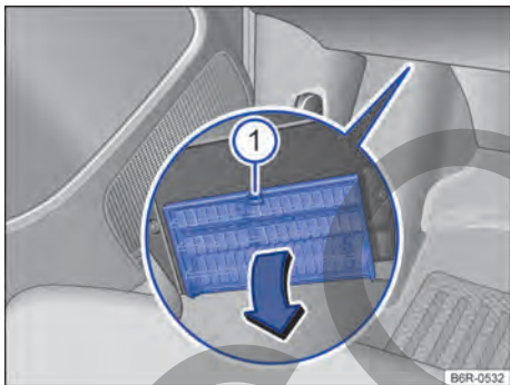
Fig. 143 En el lado del conductor debajo del panel de instrumentos: abra la cubierta de la caja de fusibles.
