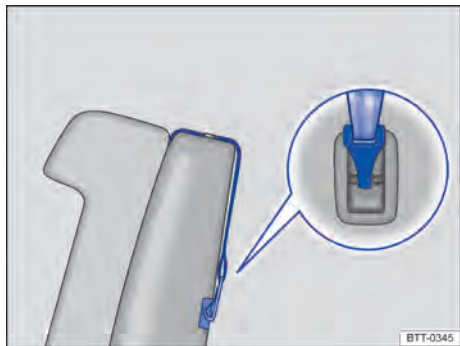
Fig. 36 Ejemplo de un cinturón de fijación superior abrochado.
