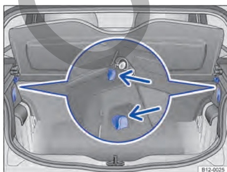
Fig. 95 En el maletero: ganchos para bolsas.
