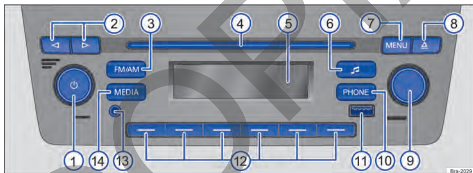
Fig. 99 Cuadro general de los mandos de la radio (variante 2).
