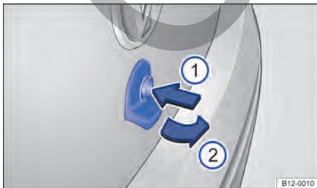
Fig. 53 Abrir el portón trasero por afuera.
