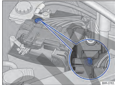
Fig. 161 En el compartimento del motor: ejemplo de posición del visor en el lado superior de la batería del vehículo.
