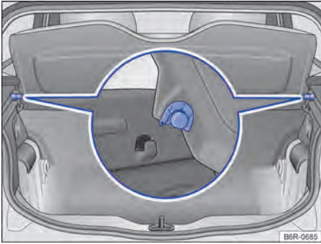
Fig. 92 En el maletero: desmontar y montar la bandeja trasera.
