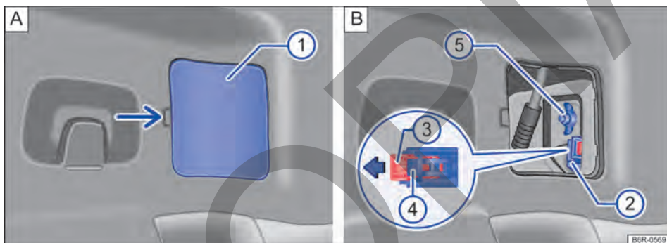
Fig. 139 Lateralmente en el compartimento de carga: A: desmontar la cubierta, B: quitar el grupo óptico trasero.
