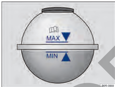
Fig. 157 En el compartimento del motor: marca en el depósito de expansión del líquido refrigerante del motor.
