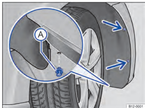
Fig. 137 En el pasarrueda delantero derecho: retirar los tornillos de fijación (flechas) y desmontar el remache de expansión (A).
