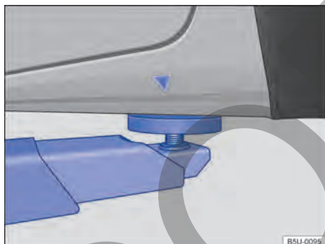
Fig. 176 Puntos de apoyo traseros para la suspensión con plataforma elevadora o con gato.
