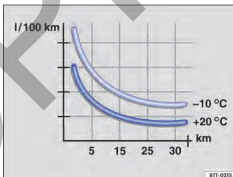
Fig. 76 Consumo de combustible en l/100 km en 2 temperaturas ambiente diferentes.
