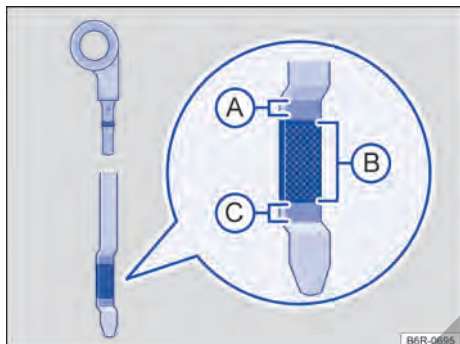
Fig. 155 Varilla de medición del aceite con marca de nivel de aceite del motor.
