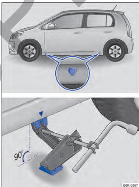
Fig. 172 Puntos de apoyo del gato y gato posicionado atrás en el lado izquierdo trasero del vehículo.
