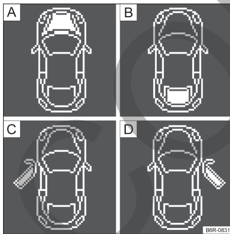
Fig. 13 En el display del instrumento combinado: indicadores de estado de la tapa del compartimento del motor, de la tapa del maletero y de las puertas.
