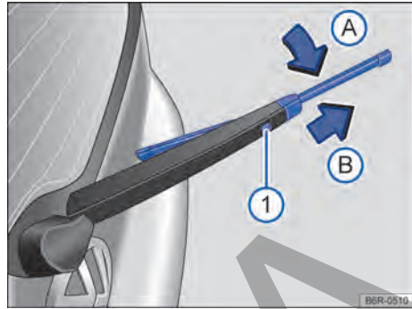
Fig. 135 Sustituir la escobilla del limpialuneta.
