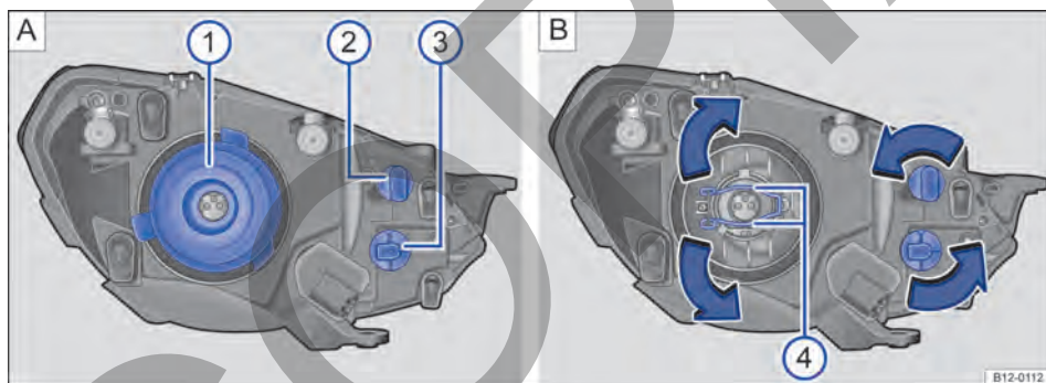
Fig. 136 En el compartimento del motor: vista trasera del faro delantero izquierdo con cubierta de goma: ① luz de cruce y luz de carretera, ② luz de posición y/o luz de conducción diurna, ③ intermitentes y bloqueo de protección ④.
