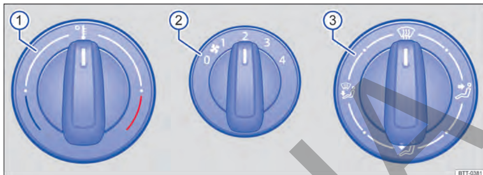
Fig. 71 En la consola central: comandos del sistema de ventilación y calefacción.
