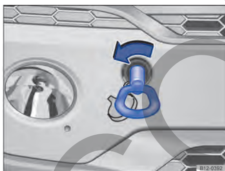
Fig. 151 En el parachoques delantero a la derecha: enrosque la argolla de remolque.
