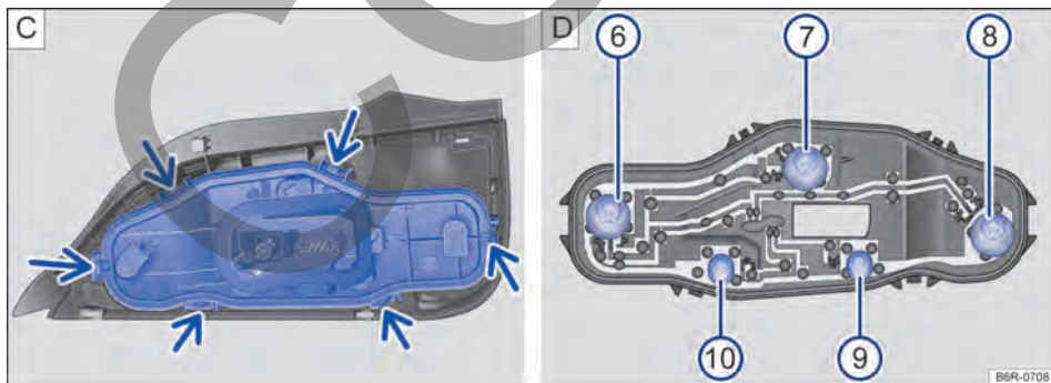
Fig. 140 Luz trasera: C: desmontar el soporte de la lámpara, D: desmontar la lámpara incandescente.
