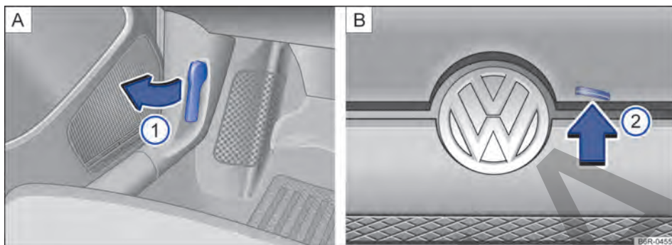
Fig. 152 A: palanca de desbloqueo en el área de los pies del lado del conductor. B: palanca de desbloqueo en la parte interna de la tapa del compartimento del motor.
