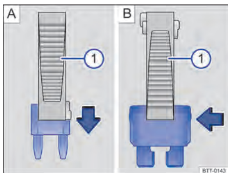
Fig. 148 Quitar o instalar un fusible con la garra de la pinza de plástico ①.
