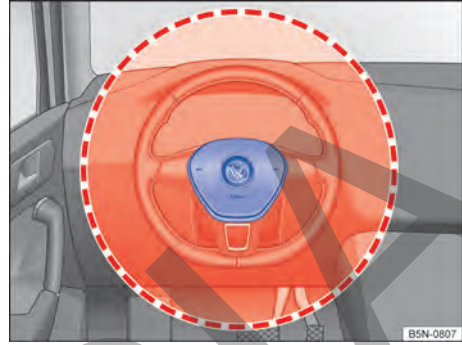
Fig. 31 En el lado del conductor: ubicación y zona de despliegue del airbag frontal del conductor.
