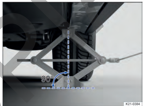
Fig. 195 Gato colocado en el lado izquierdo del vehículo, en la zona trasera (variante 2).
