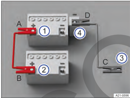
Fig. 156 Esquema para la conexión de los cables de arranque.
