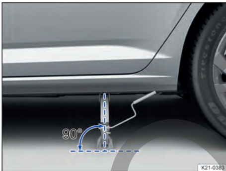
Fig. 192 Alineación correcta del gato (variante 1).
