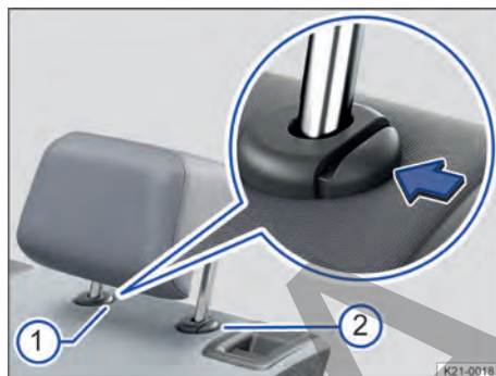
Fig. 75 Representación esquemática: desmontaje del apoyacabezas trasero central.
