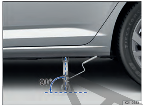
Fig. 194 Alineación correcta del gato (variante 2).
