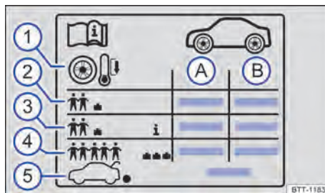
Fig. 179 Símbolos en el adhesivo de la presión de los neumáticos.
