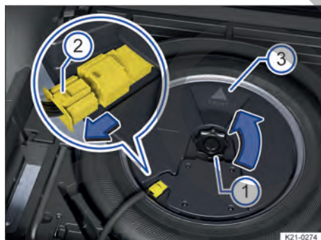
Fig. 188 En el maletero: desmontar el subwoofer.
