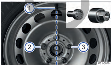
Fig. 187 Cambio de rueda: válvula del neumático (1) y lugares de montaje del tornillo de rueda antirrobo (2) o (3).
