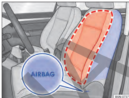
Fig. 36 En el lateral de ambos asientos delanteros: ubicación y zona de despliegue del airbag lateral.
