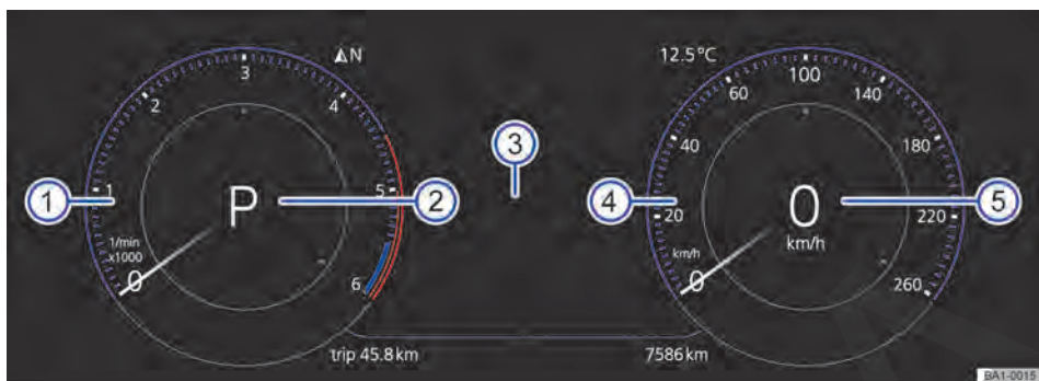
Fig. 9 Cuadro de instrumentos digital Pro en el tablero de instrumentos (representación esquemática).
