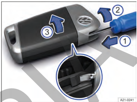
Fig. 52 Llave del vehículo: abrir la tapa del compartimento de la pila.
