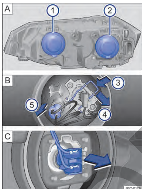
Fig. 125 En el compartimento del motor: ① farol alto y luz de posición y ② farol bajo.
