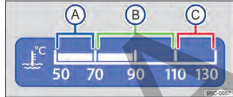
Fig. 15 Indicador de temperatura del líquido refrigerante del motor en el instrumentos combinado analógico (variante 1): (A) zona fría; (B) zona normal; (C) zona de alerta.
