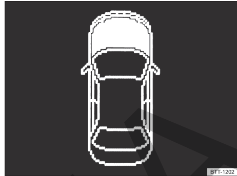
Fig. 143 En el display del instrumento combinado: tapa del compartimento del motor abierta o cerrada incorrectamente (representación esquemática).
