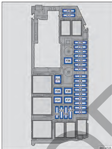
Fig. 136 En el compartimento del motor: disposición de los fusibles.
