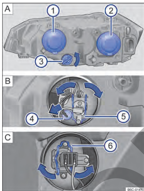
Fig. 127 En el compartimento del motor: ① farol alto y luz de posición, ② farol bajo y ③ indicador de dirección.
