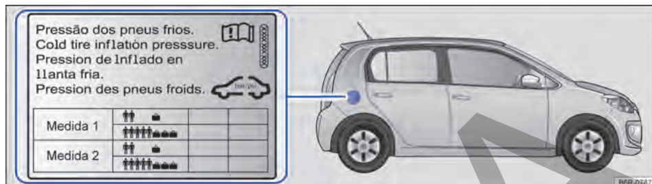
Fig. 131 En la parte interior de la portezuela del depósito de combustible: etiqueta con la presión de los neumáticos.
