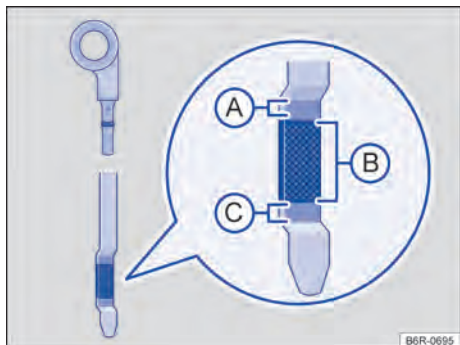
Fig. 122 Varilla de medición del aceite con marca de nivel de aceite del motor.
