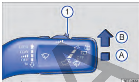
Fig. 64 Al lado del volante: palanca de los limpiavidrios: regular la sensibilidad del sensor de lluvia ①.
