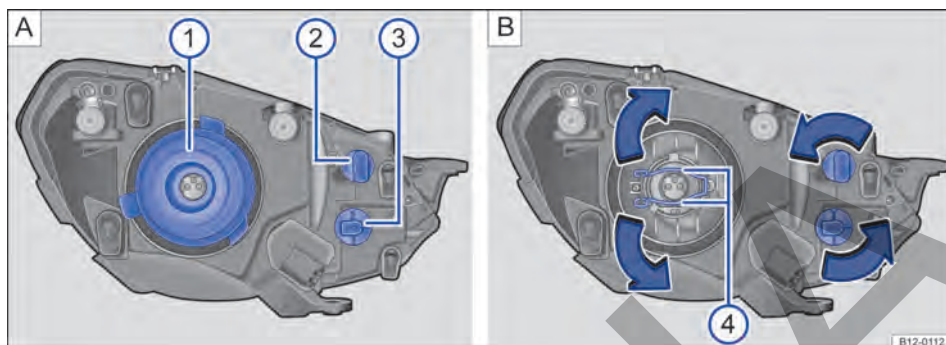
Fig. 103 En el compartimento del motor: vista trasera del farol delantero izquierdo con cubierta de goma: ① farol bajo y farol alto, ② luz de posición y/o luz de conducción diurna, ③ indicadores de dirección y bloqueo de protección ④.
