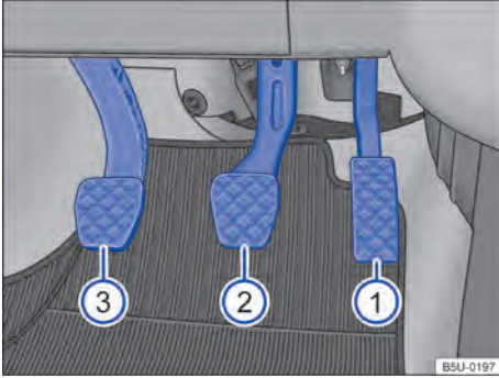
Fig. 74 En el área para los pies: pedales
