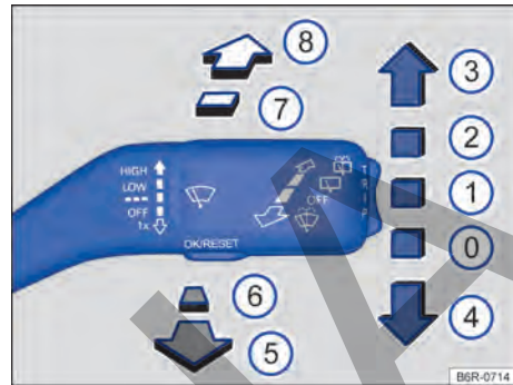
Fig. 63 Manejo de los limpiaparabrisas / lavaparabrisas y del limpiaventa / lavaluneta.
