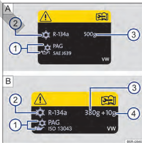
Fig. 146 (A): Información del aire acondicionado - motor MPI. (B) Información del aire acondicionado - motor TSI.
