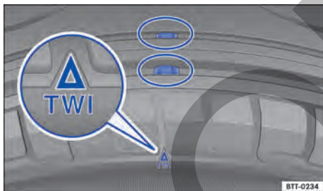
Fig. 132 Perfil del neumático: indicadores de desgaste.
