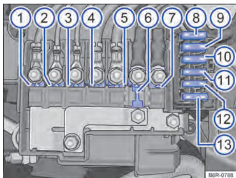
Fig. 113 Caja de fusibles.
