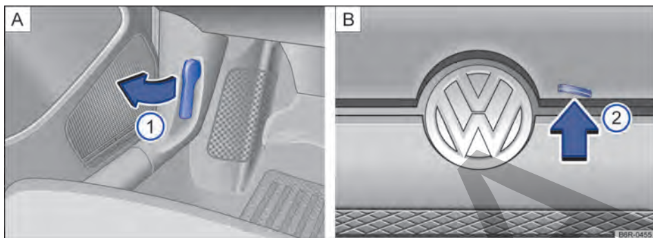
Fig. 119 A: palanca de desbloqueo en el área de los pies del lado del conductor. B: palanca de desbloqueo en la parte interna de la tapa del compartimento del motor.
