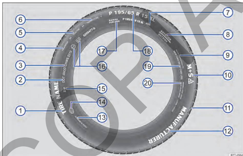
Fig. 134 Inscripción de los neumáticos internacional (ejemplo).
