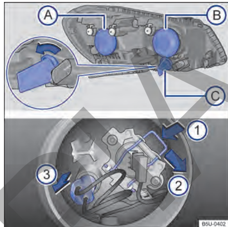
Fig. 175 En el compartimento del motor: vista trasera del faro delantero con cubierta de goma (lado izquierdo de la ilustración) - A faro bajo B faro alto y luz de posición y C indicador de dirección. Vista trasera del faro delantero sin cubierta de goma (lado derecho de la ilustración): 1 resorte de bloqueo de la lámpara incandescente del faro y 2 luz de posición.
