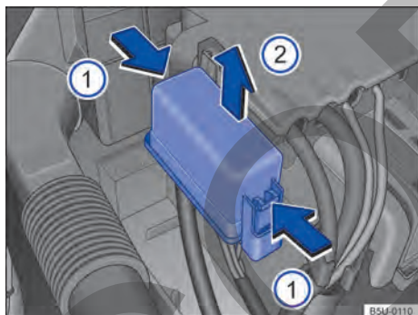
Fig. 184 En el compartimiento del motor: cobertura de la caja de fusibles.
