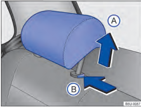
Fig. 59 Apoyacabezas traseros: desinstalar.
