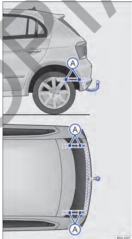
Fig. 166 Puntos de fijación para el montaje posterior de un enganche para remolque. ▶
