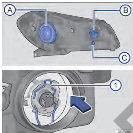
Fig. 173 En el compartimento del motor: vista trasera del farol delantero con cubierta de goma (lado izquierdo de la ilustración): A farol bajo / alto B indicadores de dirección y C luz de posición. Vista trasera del farol delantero sin cubierta de goma (lado derecho de la ilustración): 1 resorte de bloqueo de la lámpara incandescente del farol bajo/farol alto.
