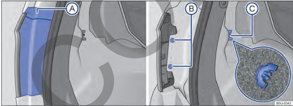
Fig. 178 En el maletero: desmontar la cubierta, retirar los dos tornillos de fijación y retirar el tornillo mariposa (fragmento ampliado).
