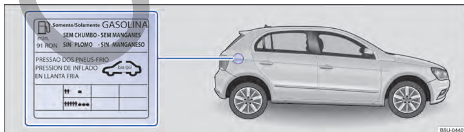
Fig. 202 En la parte interior de la portezuela del depósito de combustible: etiqueta con la presión de los neumáticos.
