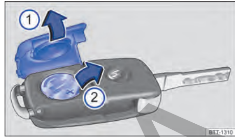
Fig. 44 Llave del vehículo con comando remoto: ① Abrir la tapa del alojamiento de la batería. ② Desmontar la batería.
