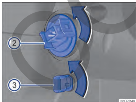
Fig. 174 En el compartimento del motor: vista trasera del farol delantero 2 indicadores de dirección y 3 luz de posición.
