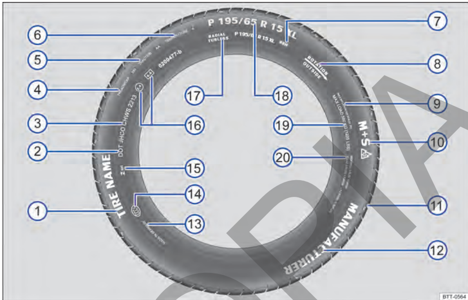
Fig. 205 Inscripción de los neumáticos internacional (ejemplo).
