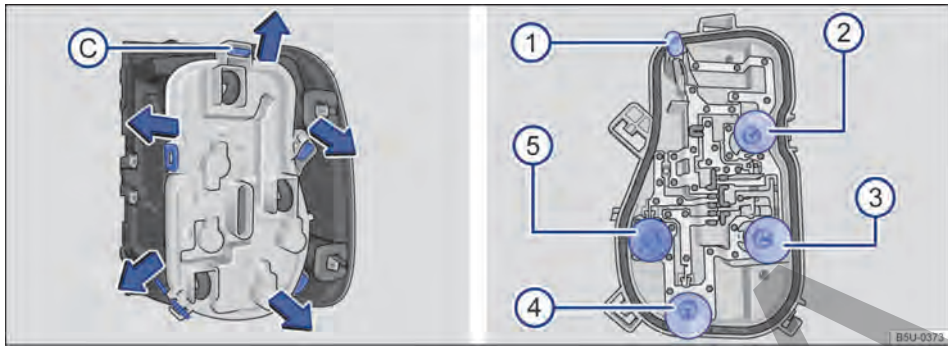
Fig. 183 Luz trasera: C desmontar el portalámparas y ①, ②, ③, ④ y ⑤ desmontar las bombillas.
