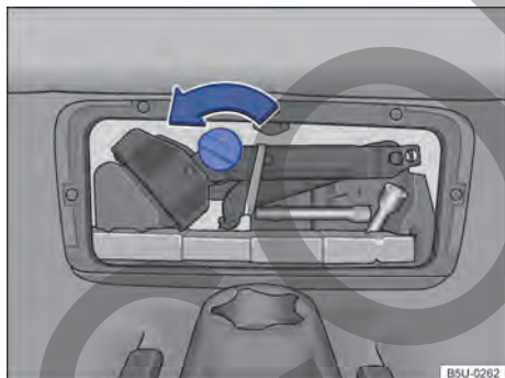
Fig. 172 Palanca de fijación de caja de herramientas de a bordo.
