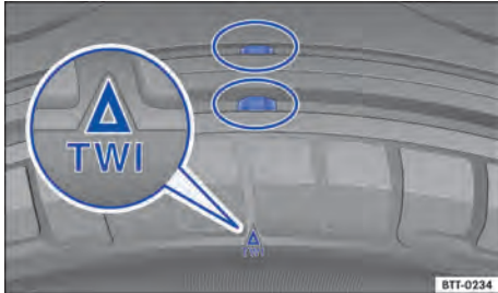
Fig. 209 Perfil del neumático: indicadores de desgaste.
