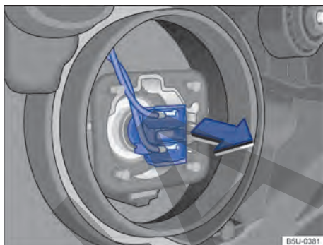
Fig. 178 Acceso a la bombilla del farol bajo.
