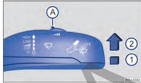
Fig. 70 Palanca de los limpiaparabrisas: ajustar la sensibilidad del sensor de lluvia (A).
