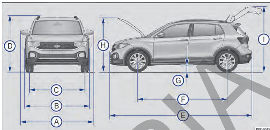
Fig. 248 Dimensiones.
