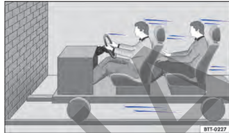
Fig. 25 Un vehículo con los ocupantes sin cinturones de seguridad está camino a chocar contra un muro.
