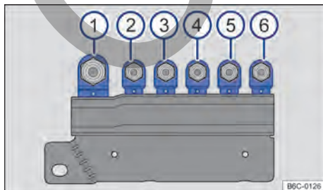
Fig. 212 En el compartimento del motor encima de la batería: disposición de los fusibles.
