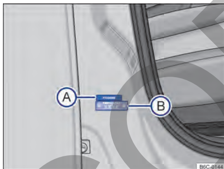
Fig. 245 En el área inferior de la columna de la puerta delantera derecha: etiqueta con el número de identificación del vehículo parcial (VIS) (A) y la placa del año de fabricación (B).
