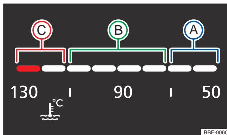
Fig. 17 Indicador de temperatura del líquido refrigerante del motor en el instrumento combinado digital (variante 2): A zona fría; B zona normal; C zona de alerta.
