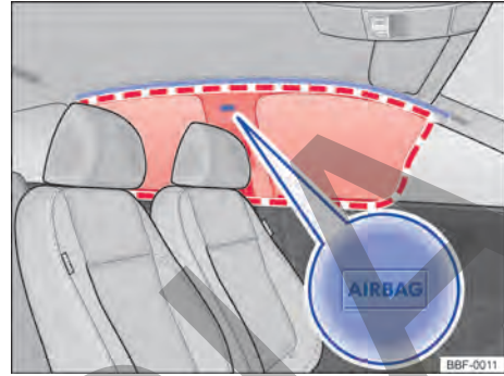
Fig. 41 En el lado izquierdo del vehículo: ubicación de montaje y área de expansión del airbag para cabeza.
