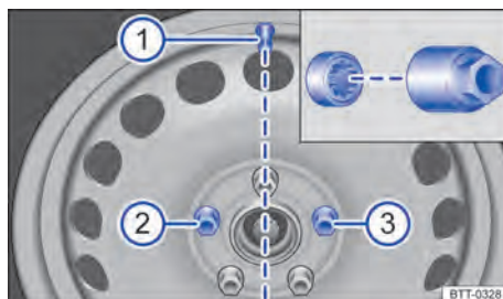
Fig. 237 Cambio de rueda: válvula del neumático ① y posición de montaje del tornillo de la rueda anti-robbo ② o ③. ▶
