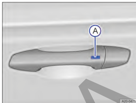
Fig. 55 En la manija de la puerta: tecla para desbloquear y bloquear.
