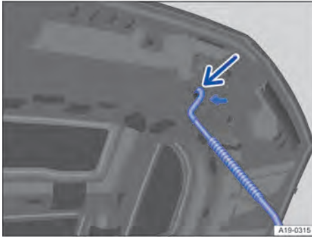
Fig. 168 En el capó delantero: alojamiento de la varilla de sujeción del capó.
