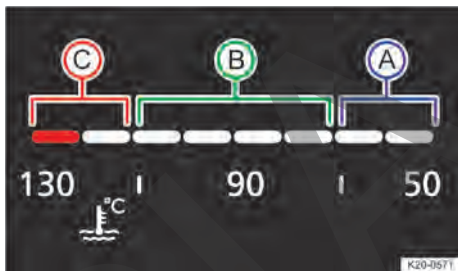
Fig. 18 Indicador de temperatura del líquido refrigerante del motor en el cuadro de instrumentos digital, versión Basic (representación esquemática).
