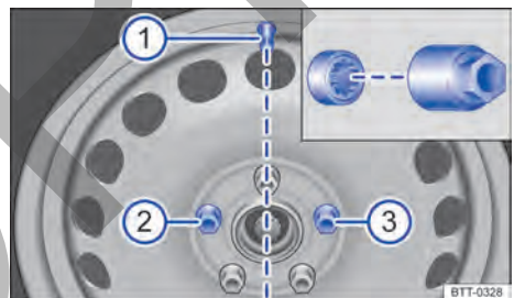
Fig. 199 Cambio de rueda: válvula del neumático ① y posición de montaje del tornillo de la rueda anti-robo ② o ③.
