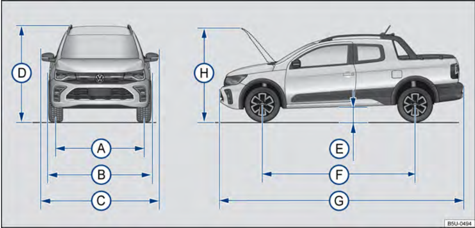
Fig. 178 Dimensiones.
