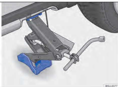
Fig. 171 Puntos de apoyo del gato y gato colocado en el lado izquierdo trasero del vehículo - vehículos con estribos exteriores.
