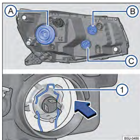
Fig. 135 En el vano motor: vista trasera del faro delantero con cubierta de goma (lado izquierdo de la ilustración) - (A) luz de cruce / luz de carretera (B) luz de posición y (C) indicadores de dirección. Vista trasera del farol delantero sin cubierta de goma (lado derecho de la ilustración): ① resorte de bloqueo de la lámpara incandescente del farol bajo/farol alto.
