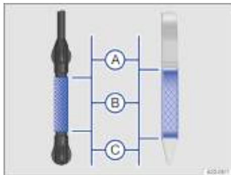
Fig. 174 Marcas del nivel de aceite del motor en la varilla de medición del nivel de aceite (variantes).
