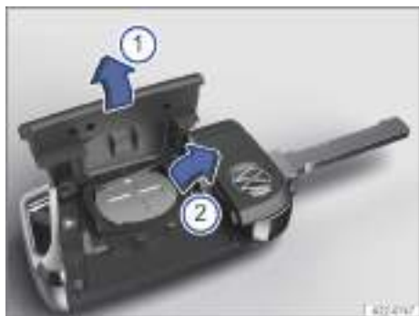
Fig. 41 Llave del vehículo: cambiar la pila de botón (representación esquemática).
