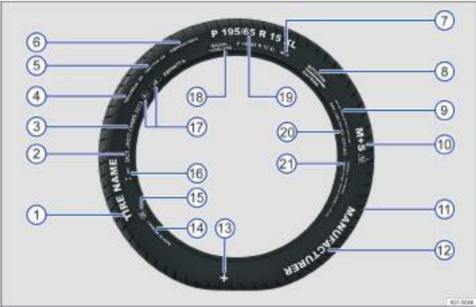
Fig. 197 Inscripciones internacionales en los neumáticos.
