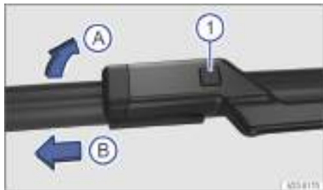
Fig. 151 Cambiar las escobillas limpiacristales del parabrisas.
