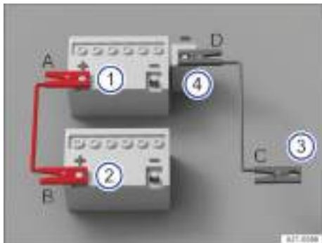
Fig. 161 Esquema para la conexión de los cables de arranque.
