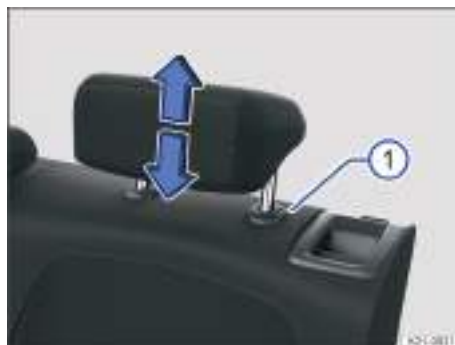
Fig. 64 Ajuste de los apoyacabezas traseros (representación esquemática).
