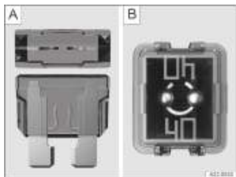
Fig. 158 Fusible fundido (representación esquemática).
