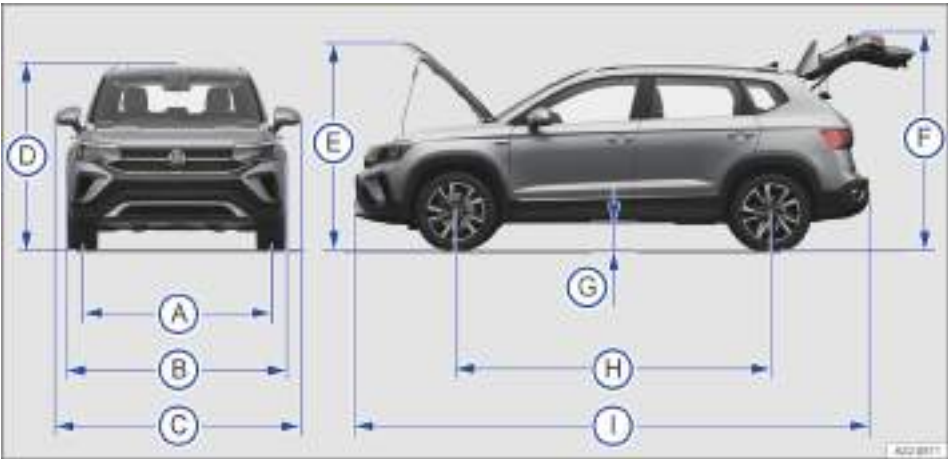
Fig. 275 Medidas del vehículo.
