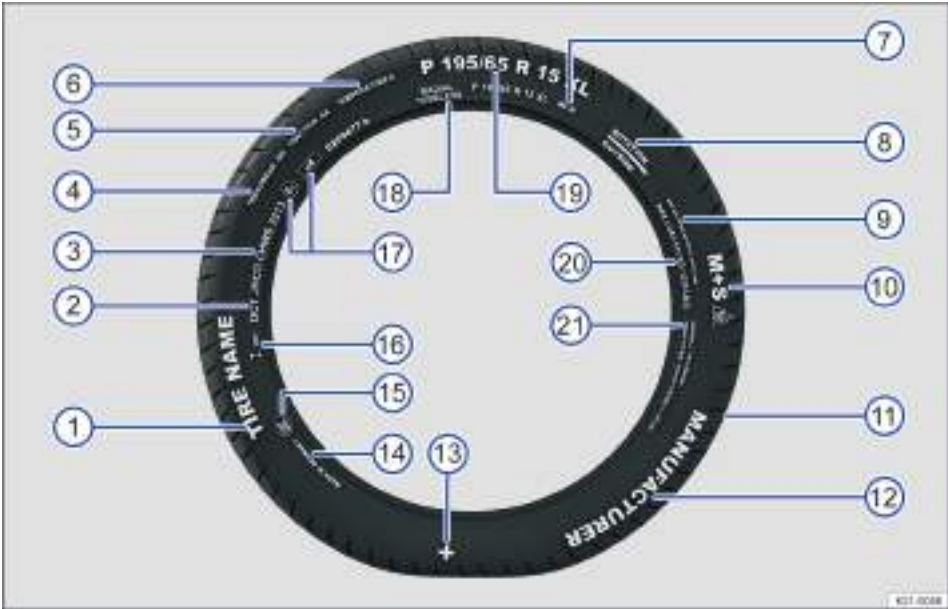
Fig. 207 Inscripciones internacionales en los neumáticos.
