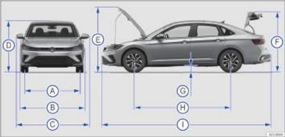
Fig. 286 Medidas del vehículo.
