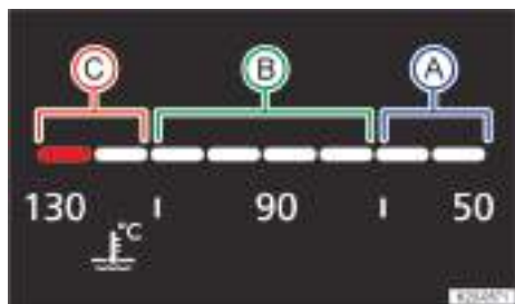
Fig. 18 En el cuadro de instrumentos digital Basic: indicador de la temperatura del líquido refrigerante (representación esquemática).
