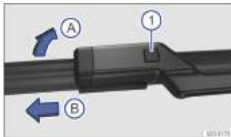
Fig. 150 Cambiar las escobillas limpiacristales del parabrisas.
