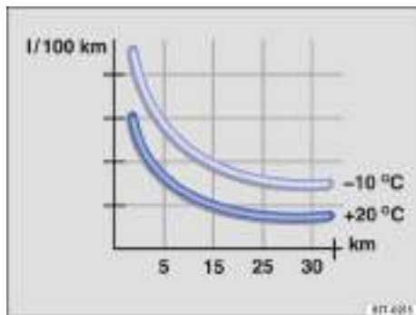
Fig. 106 Consumo de combustible en l/100 km a dos temperaturas ambiente diferentes.
