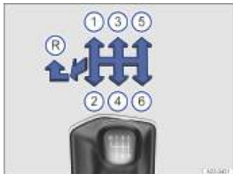
Fig. 96 Esquema de las marchas de un cambio manual de 6 marchas. En función del equipamiento, el vehículo puede estar equipado con un cambio manual de 5 marchas.
