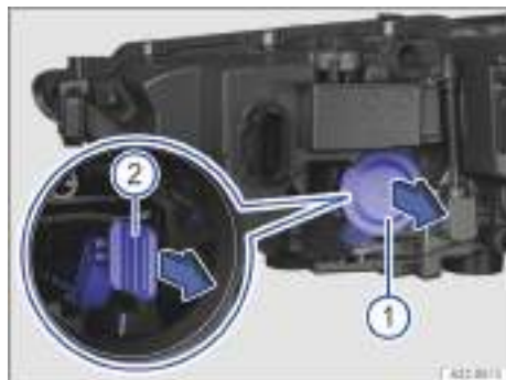
Fig. 151 En el lado derecho del vano delantero: parte trasera del faro.
