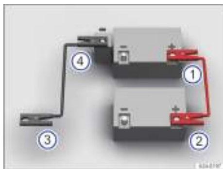
Fig. 159 Esquema para la conexión de los cables de arranque.
