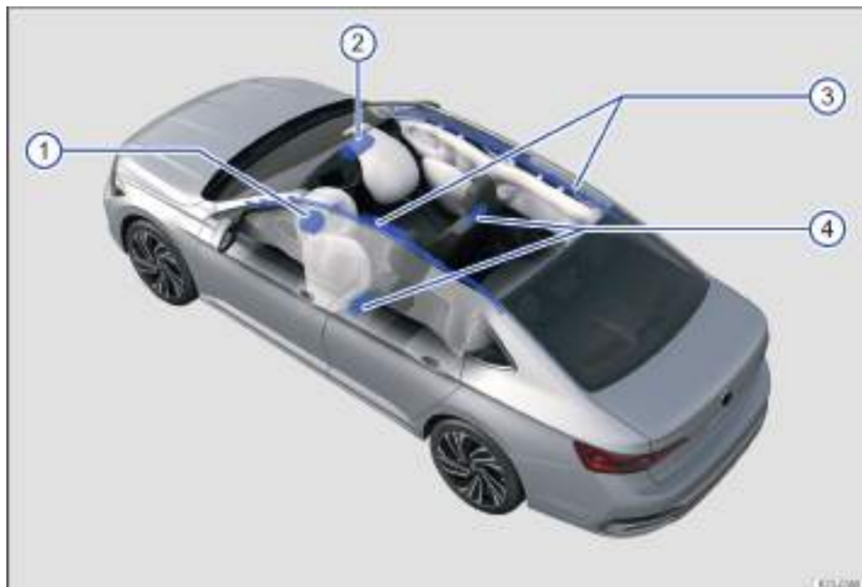
Fig. 30 Ubicaciones y zonas de despliegue de los airbags.
