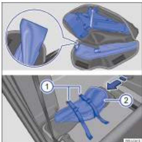
Fig. 169 Atrás del respaldo del asiento del pasajero: ② bolsas de herramientas de a bordo y ① cintas de fijación de la bolsa de las herramientas de a bordo.
