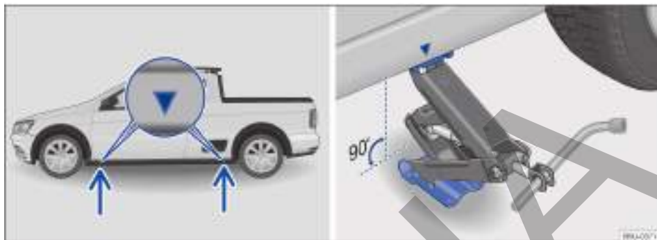
Fig. 216 Puntos de apoyo del gato y gato posicionado atrás en el lado izquierdo trasero del vehículo.
