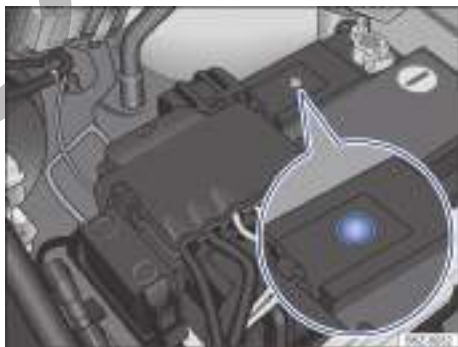
Fig. 205 En el compartimento del motor: ejemplo de posición del visor en el lado superior de la batería del vehículo.
