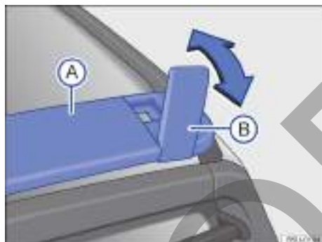
Fig. 160 En el techo: travesaño y soporte articulado.
