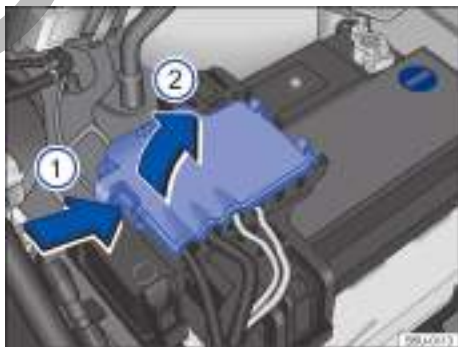
Fig. 194 Compartimento del motor: acceso al terminal positivo de la batería.
