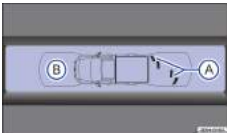
Fig. 93 Presentación del display del control de distancia de estacionamiento (display monocromático): (A) obstáculo reconocido en el segmento. (B) zona registrada delante del vehículo.
