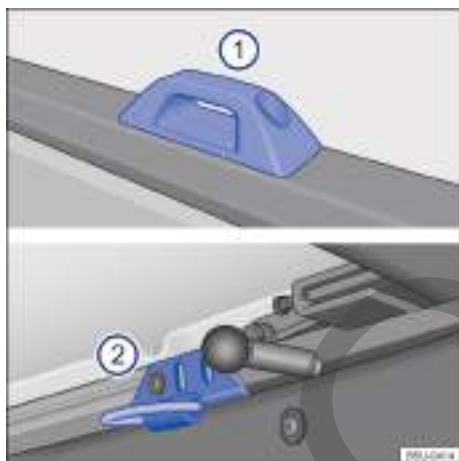
Fig. 162 En el compartimento de carga: soportes fijos ① para vehículos sin capota marítima y ② para vehículos con capota marítima.
