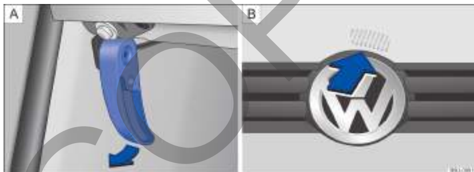
Fig. 196 [A] Palanca de desbloqueo de la tapa del compartimento del motor en la zona reposapiés del conductor. [B] Palanca de desbloqueo en la parte interior de la tapa del compartimento del motor.
