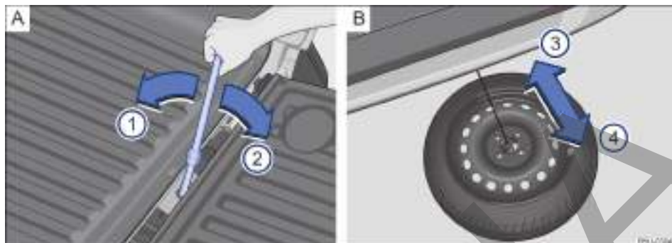
Fig. 210 A) En el compartimento de carga: acceso a la rueda de emergencia. B) Debajo del vehículo: rueda de emergencia totalmente en el piso y extracción de debajo del vehículo.
