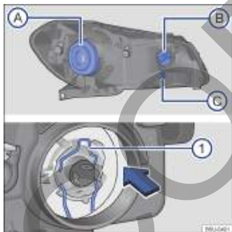
Fig. 175 En el compartimento del motor: vista trasera del farol delantero con cubierta de goma (lado izquierdo de la ilustración): A farol bajo / alto B indicadores de dirección y C luz de posición. Vista trasera del farol delantero sin cubierta de goma (lado derecho de la ilustración): 1 resorte de bloqueo de la lámpara incandescente del farol bajo/farol alto.
