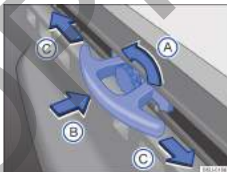
Fig. 164 En el compartimento de carga: soporte deslizante para vehículos con capota marítima.
