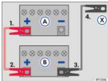
Fig. 195 Esquema para la conexión de los cables auxiliares de arranque: batería del vehículo descargada (A) y batería del vehículo que provee la corriente (B).
