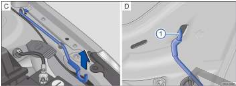
Fig. 197 [C] Varilla de sujeción de la tapa del compartimento del motor. [D] Tapa del compartimento del motor apoyada en la varilla de sujeción.
