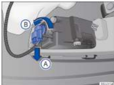
Fig. 179 Detrás del paragolpes delantero: acceso a la lámpara incandescente del farol de neblina.
