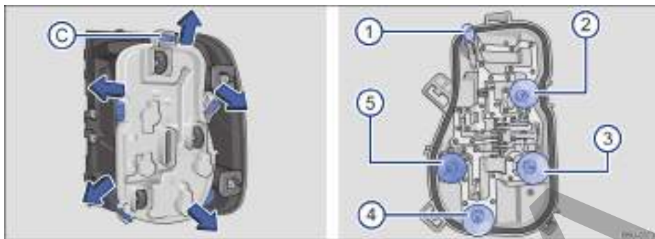
Fig. 183 Luz trasera: C desmontar el portalámparas y 1, 2, 3, 4 y 5 desmontar las bombillas.
