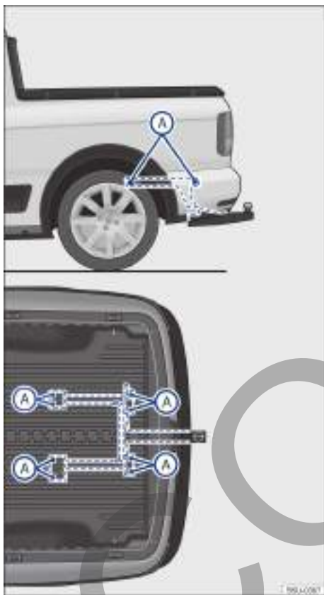
Fig. 167 Puntos de fijación para el montaje posterior de un enganche para remolque.
