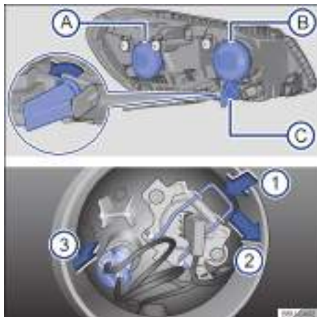
Fig. 178 Acceso a la bombilla del farol bajo.
