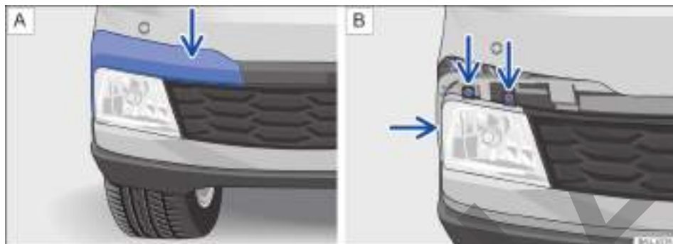
Fig. 180 En el paragolpes delantero: A desinstalar la moldura del farol de neblina y B retirar los tornillos del farol de neblina.
