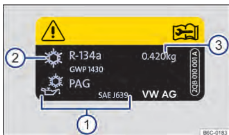
Fig. 212 Información del aire acondicionado
