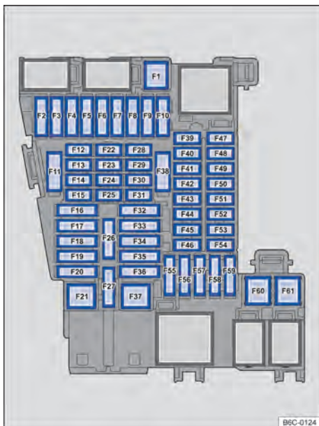
Fig. 179 En el panel de instrumentos: disposición de los fusibles.
