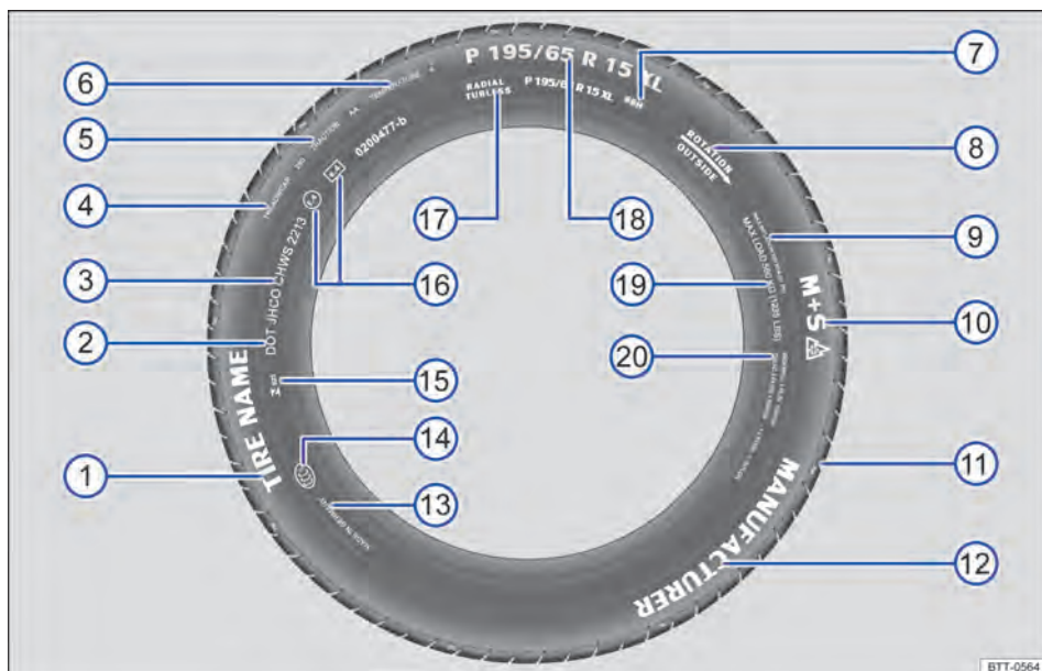
Fig. 203 Inscripción de los neumáticos internacional (ejemplo).
