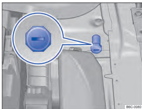
Fig. 185 En el compartimento del motor: punto de ayuda de arranque (punto de conexión a tierra).
