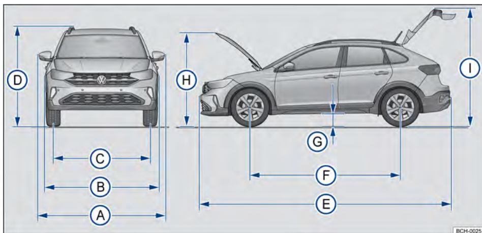
Fig. 213 Dimensiones.
