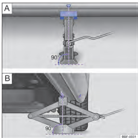
Fig. 206 Puntos de apoyo del gato y gato posicionado atrás en el lado izquierdo trasero del vehículo.
