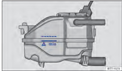
Fig. 193 En el compartimento del motor: marca en el depósito de expansión del líquido refrigerante del motor.
