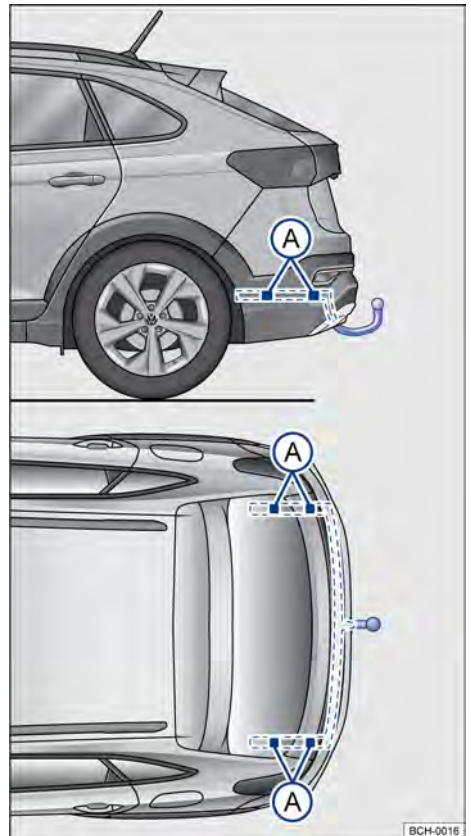
Fig. 168 Puntos de fijación para el montaje posterior de un enganche para remolque.
