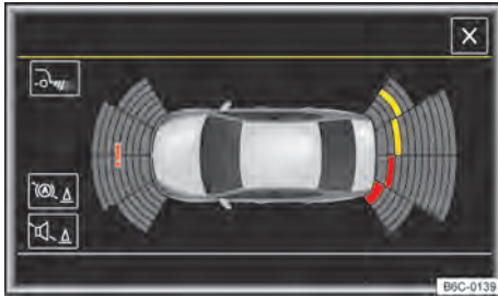
Fig. 112 Indicación no sistema de radio: modo pantalla completo. Las áreas registradas dependen de la versión del vehículo.
