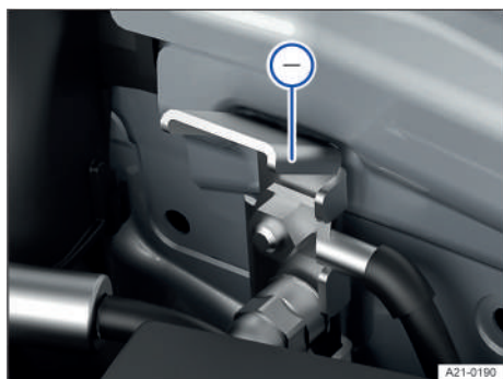
Fig. 163 En el vano delantero: toma para la ayuda de arranque, masa.
