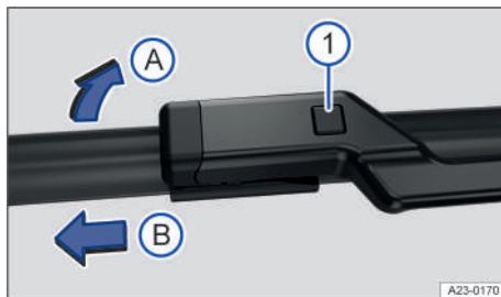
Fig. 154 Cambiar las escobillas limpiacristales del parabrisas.
