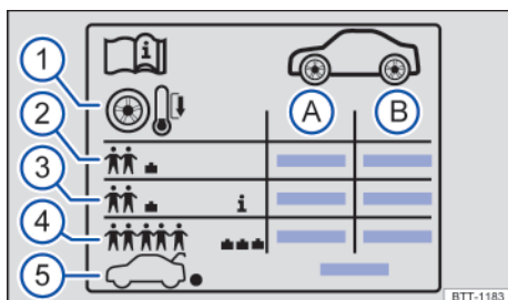
Fig. 186 Símbolos en el adhesivo de la presión de los neumáticos.
