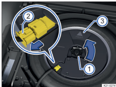
Fig. 190 En el maletero: desmontar el subwoofer (variante 2).
