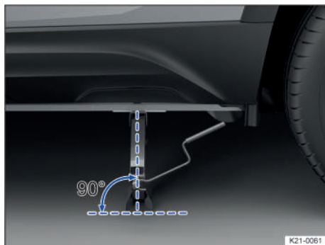
Fig. 195 Alineación correcta del gato.
