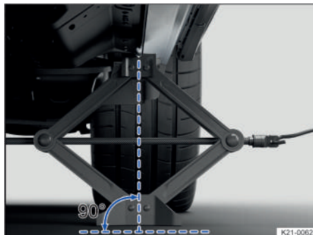
Fig. 196 En el lado izquierdo del vehículo, en la zona trasera: gato colocado.
