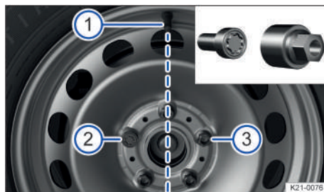
Fig. 198 Posición correcta del tornillo de rueda antirobo.
