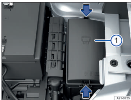
Fig. 157 En el vano delantero: caja de fusibles (representación esquemática).
