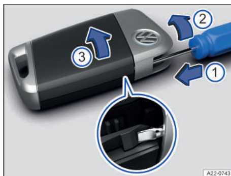
Fig. 45 Llave del vehículo: abrir la tapa del compartimento de la pila.
