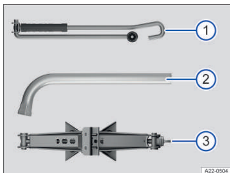
Fig. 151 Piezas adicionales de las herramientas de a bordo (representación esquemática).
