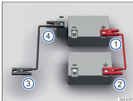
Fig. 164 Esquema para la conexión de los cables de arranque.
