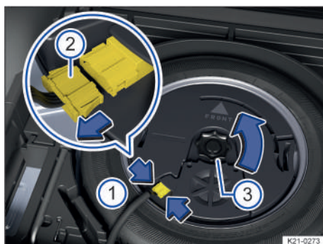
Fig. 189 En el maletero: desmontar el subwoofer (variante 1).
