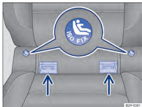
Fig. 49 En el asiento del vehículo: identificación de los puntos de anclaje inferiores de asientos para niños.
