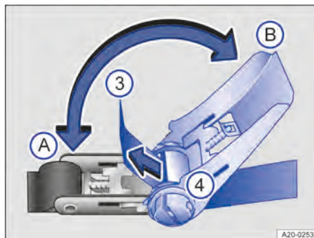
Fig. 141 Aflojar y apretar la palanca de la cinta con carraca.
