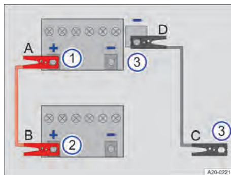
Fig. 174 Esquema para la conexión de los cables de arranque.
