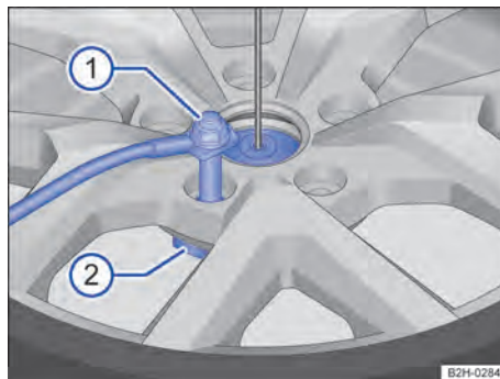
Fig. 206 Rueda de repuesto o de emergencia: soltar el tornillo de seguridad.
