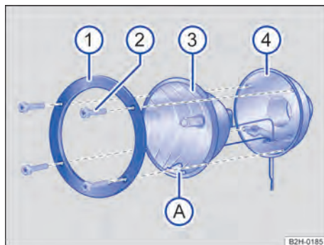
Fig. 166 Faro adicional en el techo del vehículo: desmontar el cristal.
