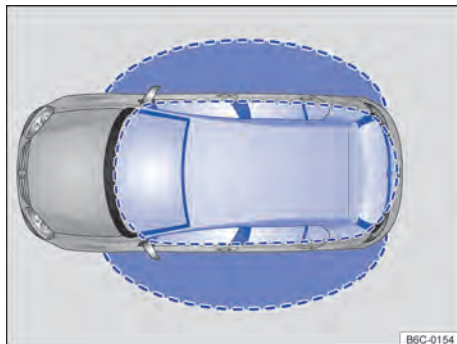
Fig. 51 Sistema "Keyless Access": áreas de aproximación.
