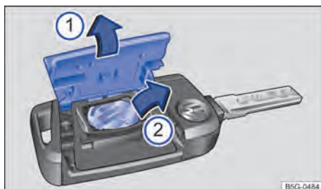
Fig. 50 Llave del vehículo: sustituir la batería.
