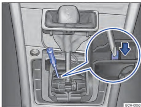
Fig. 95 Desmontar la cubierta de la palanca selectora y desbloquear el bloqueo de la palanca selectora de emergencia.
