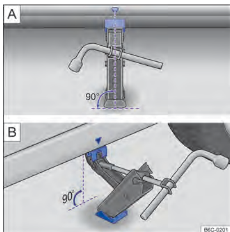
Fig. 168 Puntos de apoyo del gato y gato posicionado atrás en el lado izquierdo trasero del vehículo.
