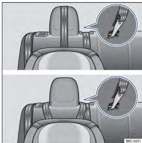
Fig. 45 En el respaldo del asiento trasero: A) colocación de la banda del cinturón en el caso de apoyacabezas no ajustables con cinturón individual Top Tether, B) colocación de la banda del cinturón en el caso de apoyacabezas no ajustables con cinturón Top Tether en forma de V.
