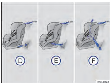
Fig. 42 En el asiento trasero: las figuras D e E muestran el principio de fijación del sistema de retención para niños en los ojales de retención inferiores y con el cinturón de fijación superior. La figura F muestra la fijación del sistema de retención para niños con el cinturón de seguridad del vehículo y con el cinturón de fijación superior.
