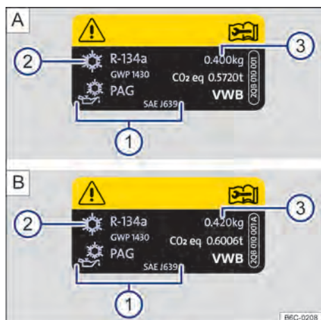
Fig. 175 A: información del aire acondicionado - motor 1.0L. B: información del aire acondicionado - motor 1.0L TSI, motor 1.4L TSI y motor 1.6L.
