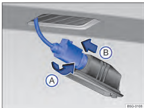
Fig. 137 Luz de la placa de licencia: desmontar el portalámparas.
