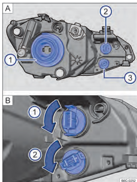
Fig. 134 En el compartimento del motor: faro delantero. ① Luz de conducción diurna y luz de posición y ② intermitente.
