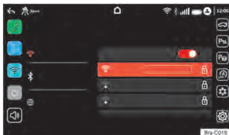
Fig. 117 Conectar Wi-Fi.
