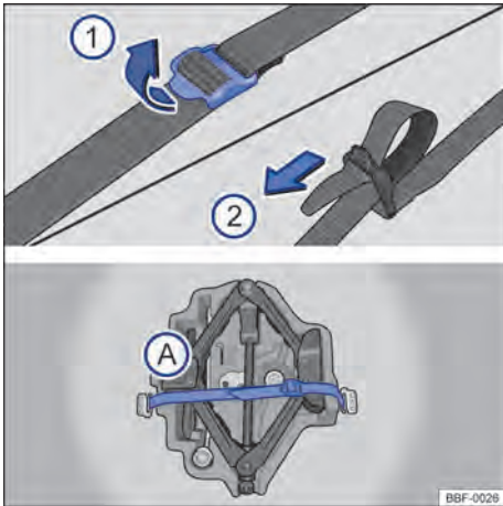
Fig. 128 En el maletero: cinta de fijación de la caja de herramientas y caja de herramientas de a bordo.
