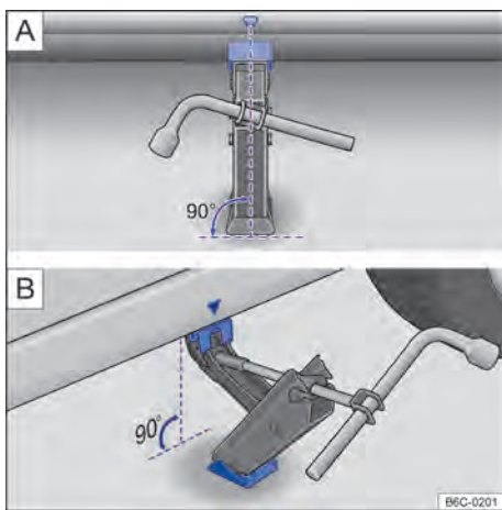
Fig. 162 Puntos de apoyo del gato y gato posicionado atrás en el lado izquierdo trasero del vehículo.
