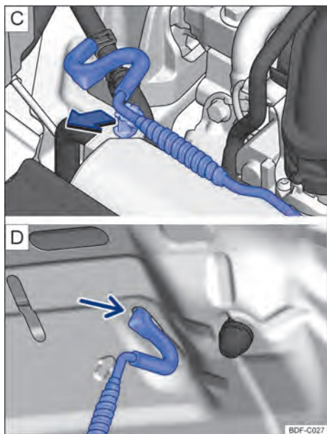
Fig. 145 [C] Varilla de sujeción de la tapa del compartimento del motor. [D] Tapa del compartimento del motor apoyada en la varilla de sujeción.
