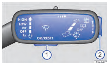
Fig. 15 Vehículos sin volante multifunción: tecla ① en la palanca del limpiacristsales para confirmación de las opciones de menú y llave ② para alternar entre los menús.
