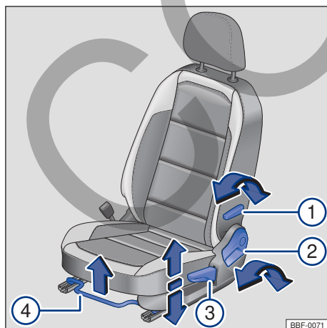
Fig. 63 En el asiento delantero: comandos.
