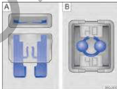
Fig. 210 Fusible quemado: A) fusible plano, B) fusible de bloqueo.
