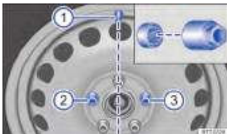
Fig. 234 Cambio de rueda: válvula del neumático ① y posición de montaje del tornillo de la rueda anti-robto ② o ③.
