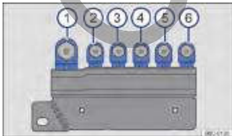
Fig. 209 En el compartimento del motor encima de la batería: disposición de los fusibles.
