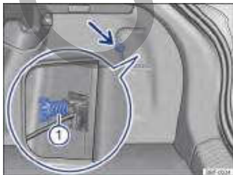
Fig. 203 En el maletero: desmontar la cubierta y retirar el tornillo mariposa ① (fragmento ampliado).
