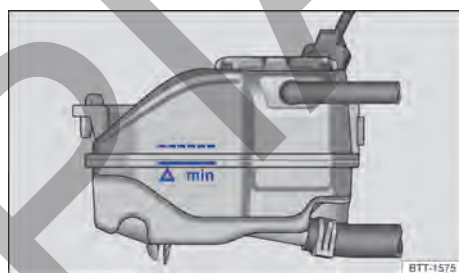
Fig. 182 En el compartimento del motor: marca en el depósito de expansión del líquido refrigerante del motor.
