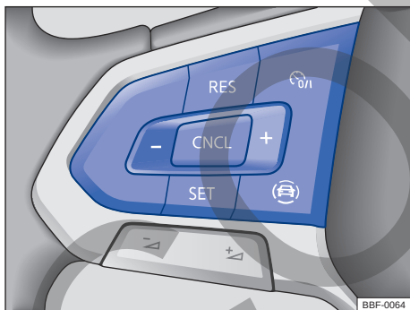
Fig. 96 Lado izquierdo del volante multifunción (variante 2): teclas para controlar el limitador de velocidad.
