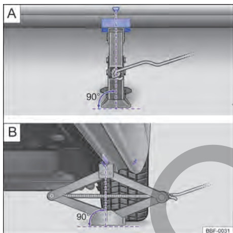
Fig. 195 Puntos de apoyo del gato y gato posicionado atrás en el lado izquierdo trasero del vehículo.
