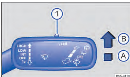
Fig. 74 A la derecha de la columna de dirección: palanca de los limpiavidrios.
