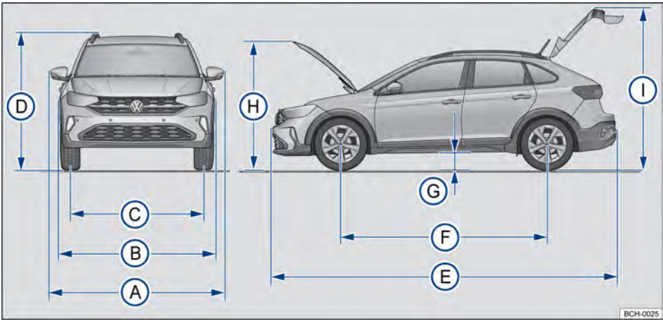
Fig. 203 Dimensiones.
