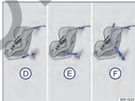
Fig. 40 En el asiento trasero: las figuras D y E muestran el principio de fijación del sistema de retención infantil en los ojalos de retención inferiores y con el cinturón de fijación superior. La figura F muestra la fijación del sistema de retención para niños con el cinturón de seguridad del vehículo y con el cinturón de fijación superior.
