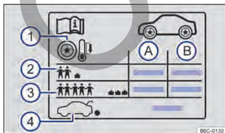
Fig. 188 Etiqueta con las presiones de los neumáticos
