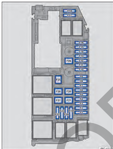
Fig. 171 En el compartimento del motor: disposición de los fusibles.
