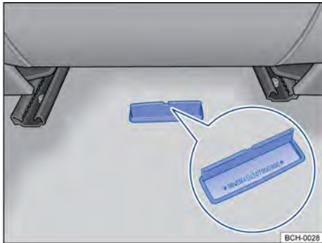
Fig. 200 Delante del asiento del pasajero trasero en el piso derecho: número de identificación del vehículo (número de bastidor).
