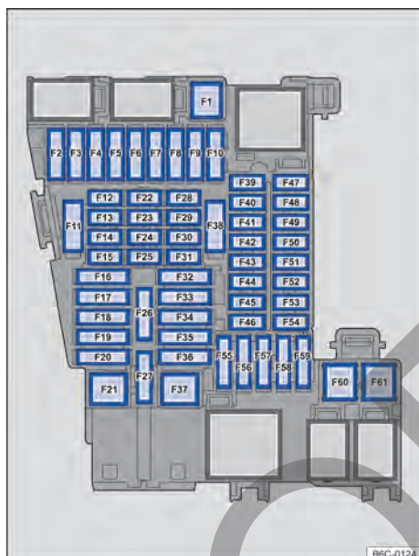
Fig. 169 En el panel de instrumentos: disposición de los fusibles.
