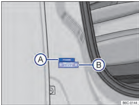
Fig. 201 En el área inferior de la columna de la puerta delantera derecha: etiqueta con el número de identificación del vehículo parcial (VIS) (A) y la placa del año de fabricación (B).
