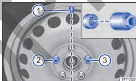
Fig. 199 Cambio de rueda: válvula del neumático ① y posición de montaje del tornillo de la rueda anti-robo ② o ③.
