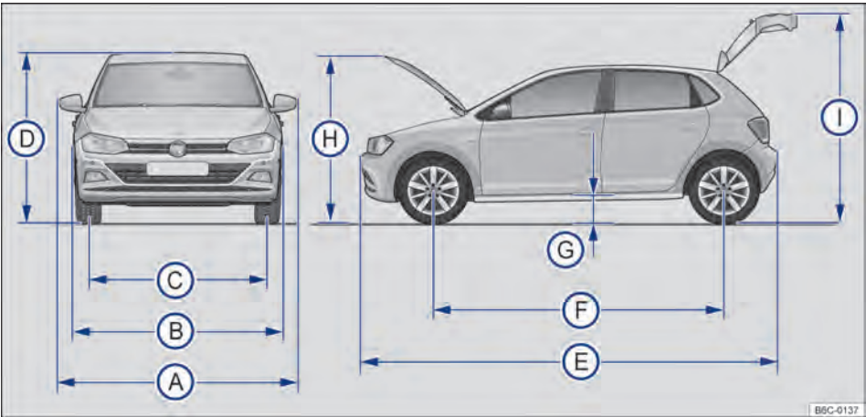
Fig. 207 Dimensiones.
