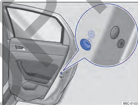
Fig. 45 En la puerta trasera (lado derecho): ubicación del seguro para niños.
