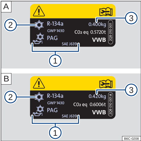
Fig. 206 [A]: Información del aire acondicionado - motor 1.0L. [B]: información del aire acondicionado - motor 1.0L TSI, motor 1.4L TSI y motor 1.6L.
