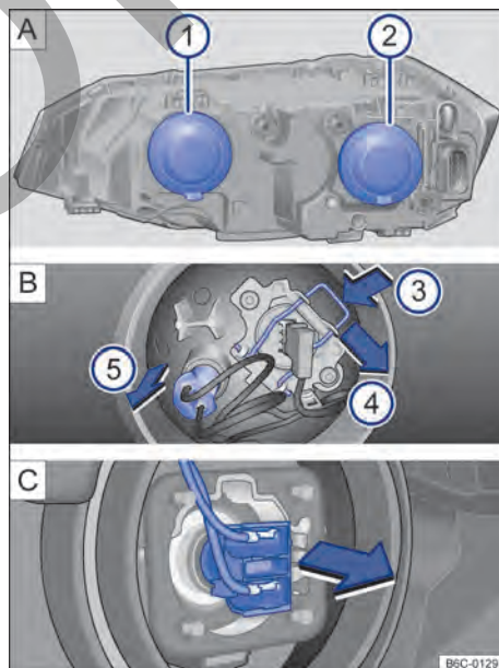
Fig. 163 En el compartimento del motor: ❶ faro alto y luz de posición y ❷ faro bajo. ▶
