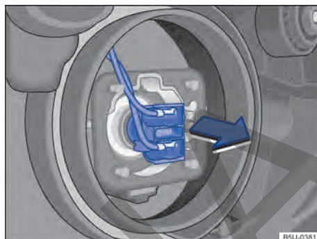
Fig. 184 Acceso a la bombilla del faro bajo.
