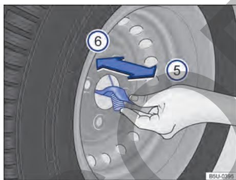
Fig. 217 En la rueda de emergencia: retirar el cable de la rueda de emergencia.
