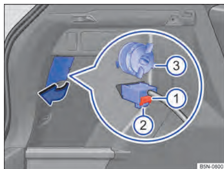
Fig. 218 Lateral del maletero: desmontaje del grupo óptico trasero.
