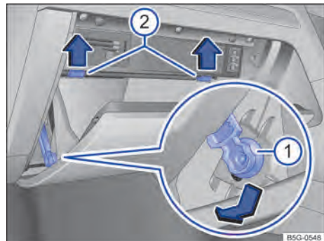
Fig. 222 En el lado del acompañante: tapa de la caja de fusibles del tablero de instrumentos (vehículos con el volante a la derecha).
