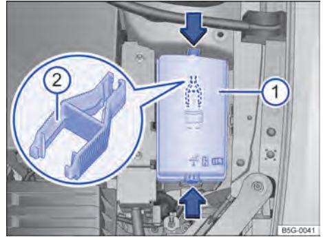
Fig. 219 En el vano motor: cubierta ① de la caja de fusibles con pinzas de plástico ②.
