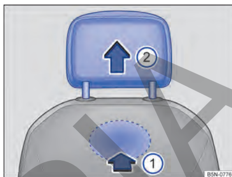
Fig. 94 Apoyacabezas delantero: desmontaje.
