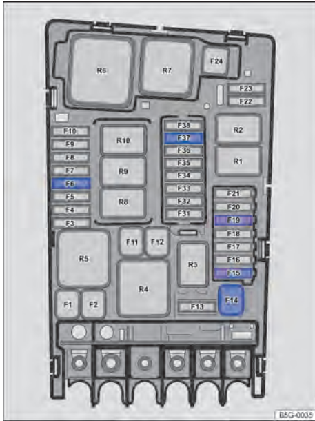
Fig. 220 En el vano motor: posiciones de los fusibles.
