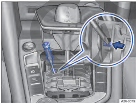
Fig. 133 Realizar un desbloqueo de emergencia de la palanca selectora (variante 1).
