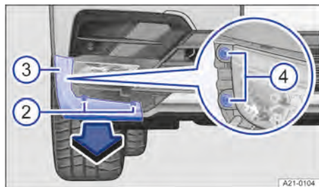
Fig. 217 En el lado derecho del paragolpes delantero R-Line: desmontar el faro antiniebla.
