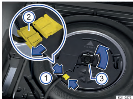
Fig. 257 En el maletero: desmontar el subwoofer (variante 1).
