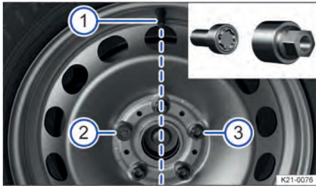
Fig. 256 Cambio de rueda: válvula del neumático ① y lugares de montaje del tornillo de rueda antirrobo ② o ③.
