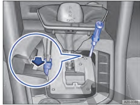
Fig. 134 Realizar un desbloqueo de emergencia de la palanca selectora (variante 2).
