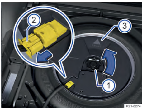
Fig. 258 En el maletero: desmontar el subwoofer (variante 2).
