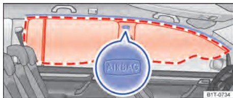
Fig. 42 En el lado izquierdo del vehículo (5 plazas): ubicación y zona de despliegue del airbag para la cabeza.
