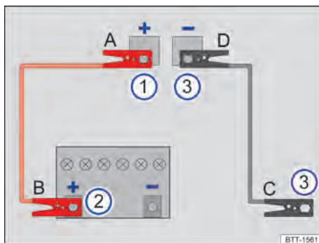
Fig. 229 Esquema para la conexión de los cables de arranque (batería de 12 voltios en el maletero).
