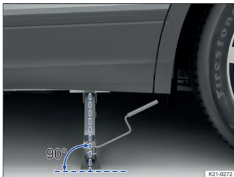
Fig. 261 Alineación correcta del gato.
