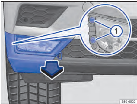
Fig. 215 En el lado derecho del paragolpes delantero: desmontaje del faro antiniebla.
