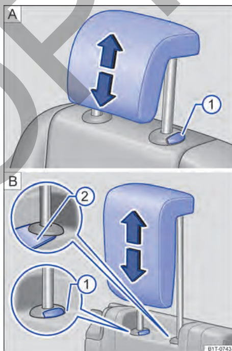
Fig. 95 Apoyacabezas trasero: desmontaje.
