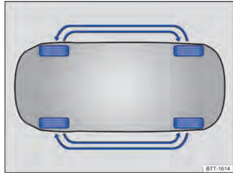
Fig. 247 Representación esquemática: esquema para el intercambio de las ruedas.
