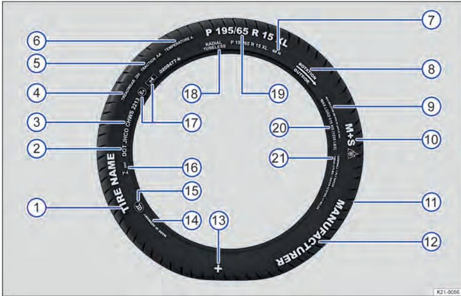
Fig. 251 Inscripciones internacionales en los neumáticos.
