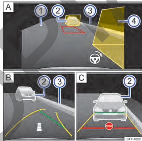
Fig. 165 Sistema de infotainment: aparcarse en línea.
