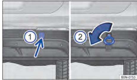
Fig. 233 En el lado derecho del paragolpes trasero: argolla de remolque enroscada.
