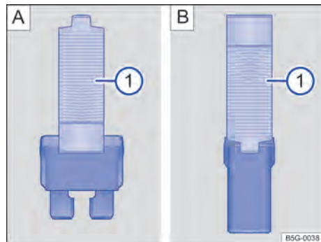
Fig. 225 Extraer o colocar un fusible con las pinzas de plástico (representación esquemática).
