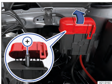
Fig. 227 En el vano motor debajo de una cubierta: toma para la ayuda de arranque (polo positivo).
