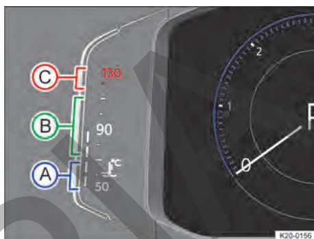
Fig. 20 Indicador de temperatura del líquido refrigerante del motor en el cuadro de instrumentos digital, versión Pro (representación esquemática).
