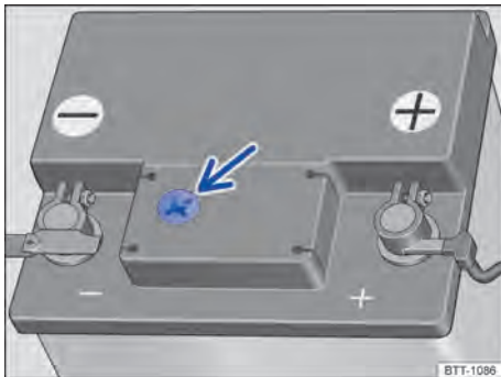
Fig. 245 Mirilla en la parte superior de la batería de 12 voltios (representación esquemática).
