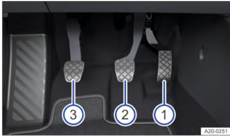
Fig. 121 En la zona reposapiés: pedales en los vehículos con cambio manual.
