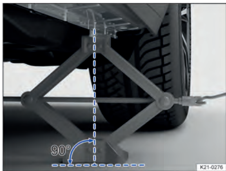
Fig. 262 Gato colocado en el lado izquierdo del vehículo, en la zona trasera.
