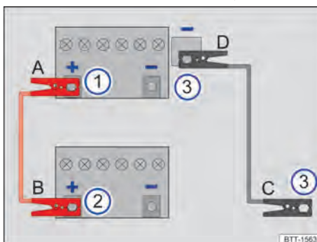
Fig. 228 Esquema para la conexión de los cables de arranque (batería de 12 voltios en el vano motor).
