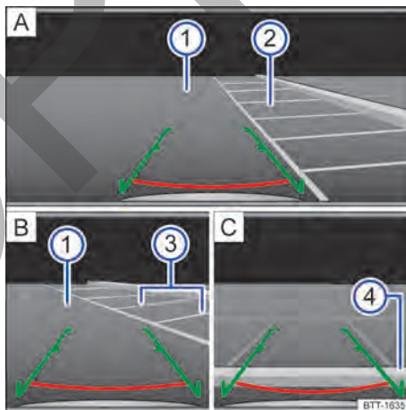
Fig. 163 Sistema de infotainment: aparcamiento con el asistente de marcha atrás.
