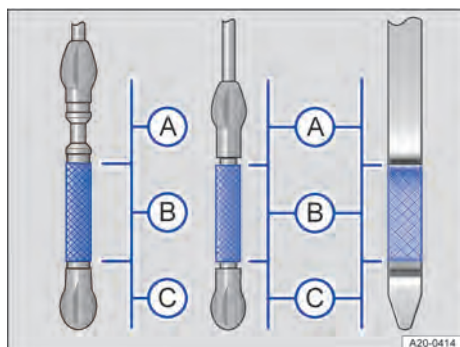
Fig. 240 Marcas del nivel de aceite del motor en la varilla de medición del nivel de aceite (variantes).
