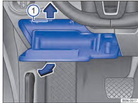
Fig. 221 Junto al volante, en el lado izquierdo: tapa de la caja de fusibles del tablero de instrumentos (vehículos con el volante a la izquierda).
