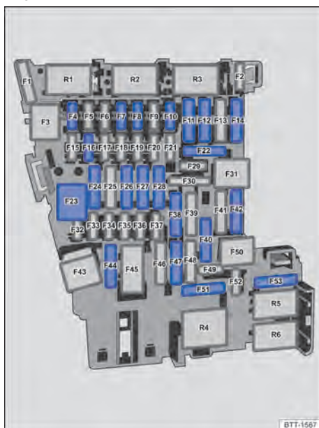
Fig. 223 En el tablero de instrumentos: asignación de fusibles.
