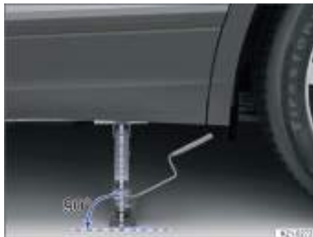
Fig. 277 Alineación correcta del gato.
