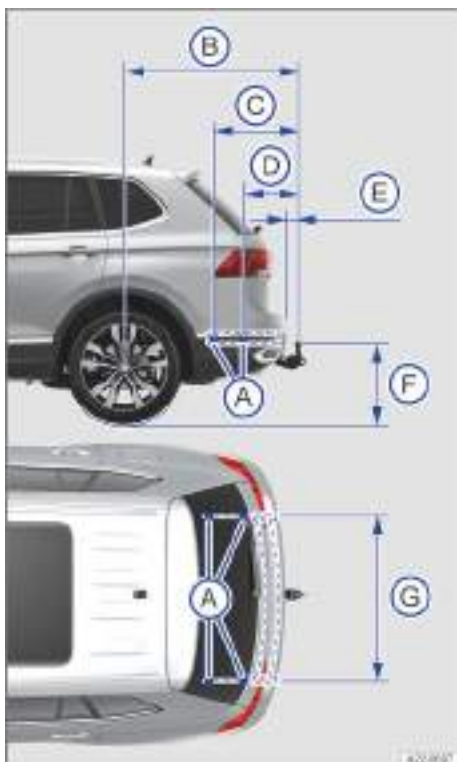
Fig. 218 Cotas y puntos de fijación para el montaje posterior de un dispositivo de remolque.
