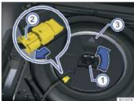
Fig. 271 Debajo del piso del maletero: desmontar el subwoofer (variante 2).
