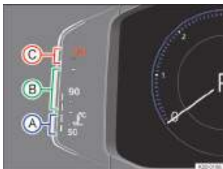
Fig. 25 En el cuadro de instrumentos digital Pro: indicador de temperatura del líquido refrigerante del motor (representación esquemática).
