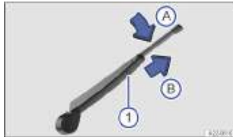
Fig. 235 Cambiar la escobilla limpiacristales de la luneta.
