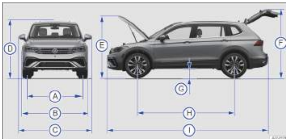
Fig. 331 Medidas del vehículo.
