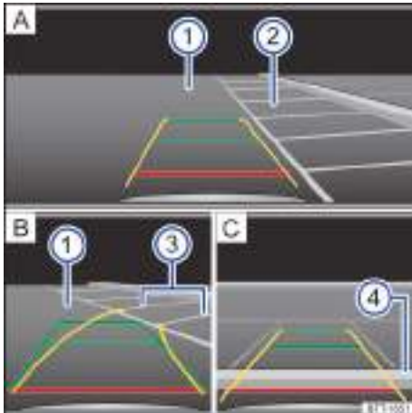
Fig. 179 Sistema de infotainment: aparcar en batería.
