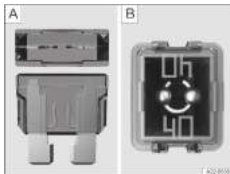
Fig. 242 Fusible fundido (representación esquemática).
