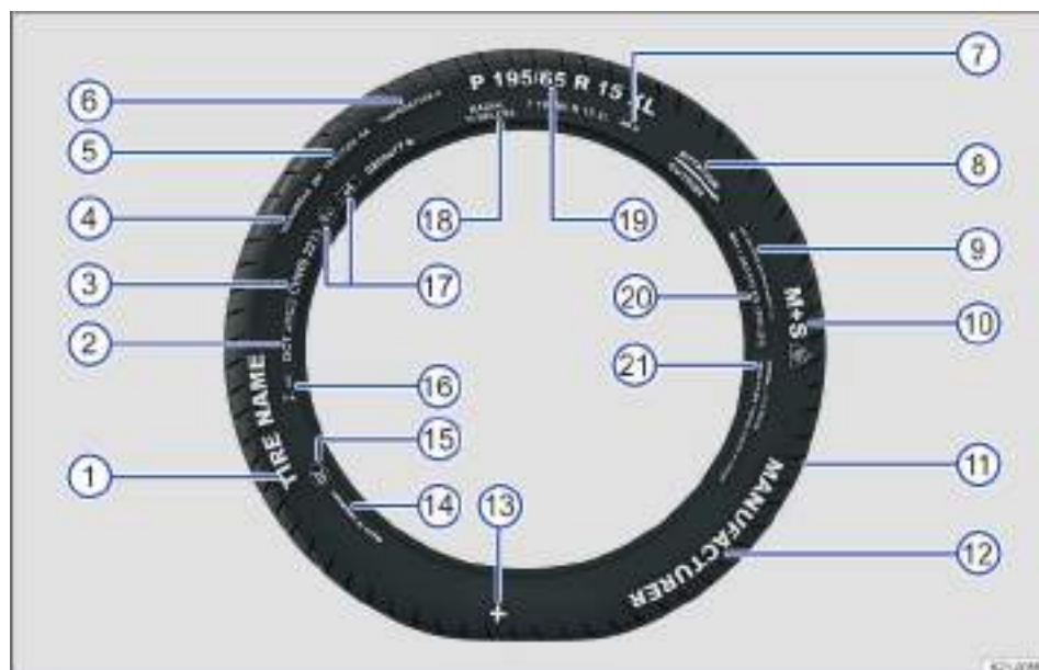
Fig. 285 Inscripciones internacionales en los neumáticos.
