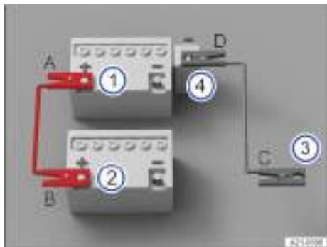
Fig. 245 Esquema para la conexión de los cables de arranque.
