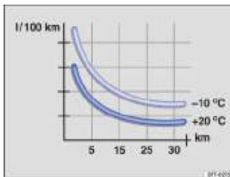
Fig. 156 Consumo de combustible en l/100 km a dos temperaturas ambiente diferentes.
