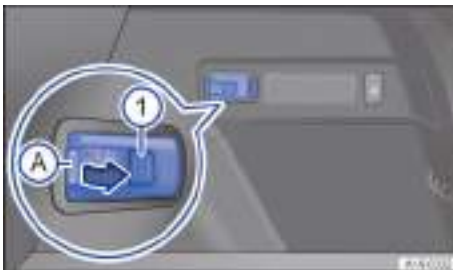
Fig. 215 En el lado derecho del maletero: unidad de iluminación extraíble.
