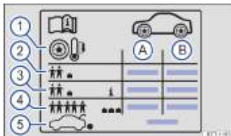
Fig. 263 Símbolos en el adhesivo de la presión de los neumáticos.
