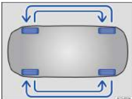
Fig. 267 Esquema para el intercambio de las ruedas (representación esquemática).
