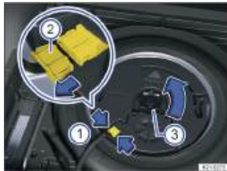
Fig. 270 Debajo del piso del maletero: desmontar el subwoofer (variante 1).
