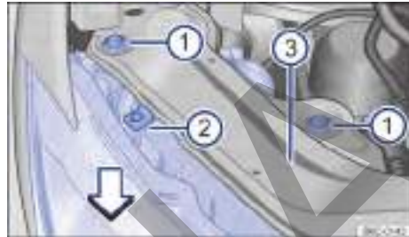
Fig. 162 En el compartimento del motor: tornillos de fijación del farol delantero.
