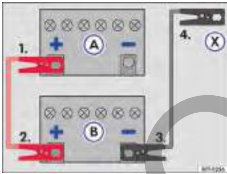
Fig. 179 Esquema para la conexión de los cables auxiliares de arranque: batería del vehículo descargada (A) y batería del vehículo que provee la corriente (B).
