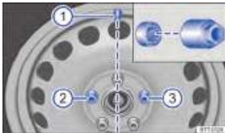
Fig. 199 Cambio de rueda: válvula del neumático ① y posición de montaje del tornillo de la rueda anti-robbo ② o ③.
