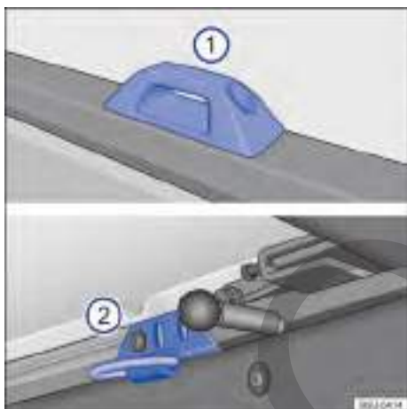
Fig. 162 En el compartimento de carga: soportes fijos 1 para vehículos sin capota marítima y 2 para vehículos con capota marítima.
