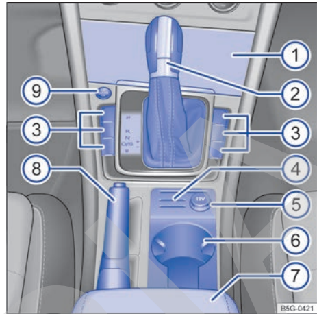
Fig. 11 Cuadro general de la parte inferior de la consola central.
