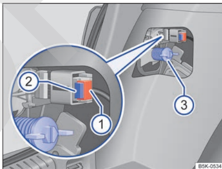
Fig. 191 Lateral del maletero: desmontaje del grupo óptico trasero. ▶
