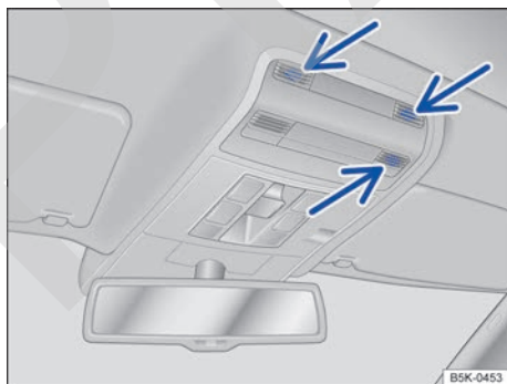
Fig. 67 En la consola del techo: sensores de la vigilancia del habitáculo (flechas).
