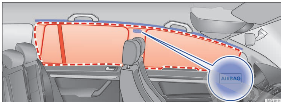
Fig. 46 En el lado izquierdo del vehículo: ubicación y zona de despliegue del airbag para la cabeza (Variant).
