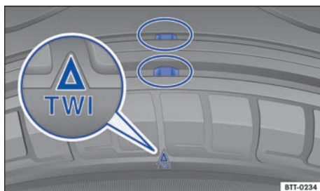
Fig. 229 Perfil del neumático: indicadores de desgaste.
