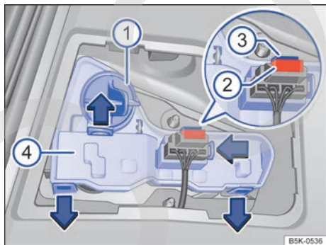
Fig. 196 En el portón del maletero: extraer el portalámparas.
