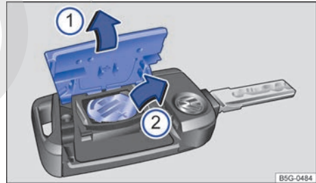
Fig. 58 Llave del vehículo: cambiar la pila de botón.
