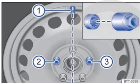
Fig. 237 Cambio de rueda: válvula del neumático ① y lugar de montaje del tornillo de rueda antirrobo ② o ③.
