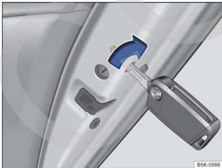
Fig. 64 En el frontal de la puerta trasera derecha: bloqueo de emergencia del vehículo con la llave de este.
