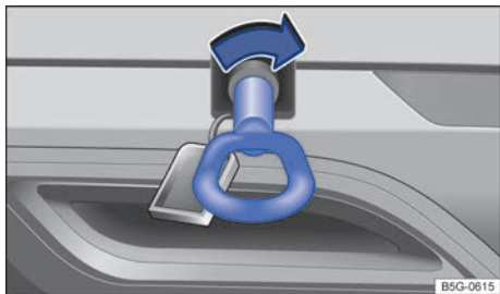
Fig. 211 En el lado derecho del paragolpes trasero: enroscar la argolla de remolque.
