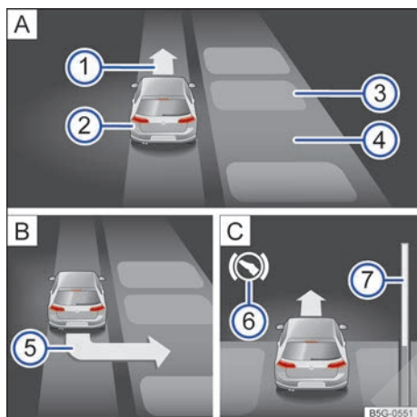
Fig. 137 En la pantalla del cuadro de instrumentos: aparcarse en batería. A Buscar un hueco de aparcamiento. B Posición para aparcarse. C Maniobrar.
