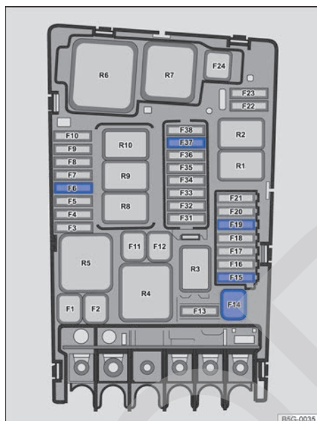
Fig. 205 En el vano motor: posiciones de los fusibles.
