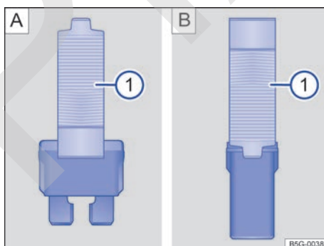
Fig. 207 Extraer o colocar el fusible con las pinzas de plástico: A Fusible enchufable plano. B Fusible tipo bloque.
