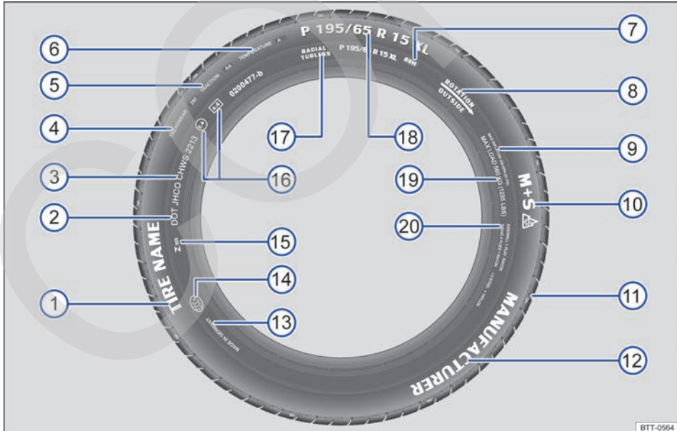
Fig. 231 Inscripciones internacionales en los neumáticos.
