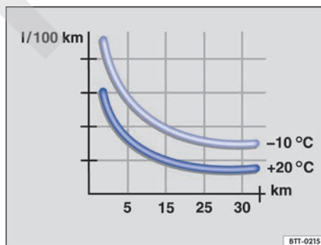
Fig. 105 Consumo de combustible en l/100 km a dos temperaturas ambiente diferentes.
