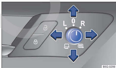
Fig. 96 En la puerta del conductor: mando giratorio de los retrovisores exteriores.
