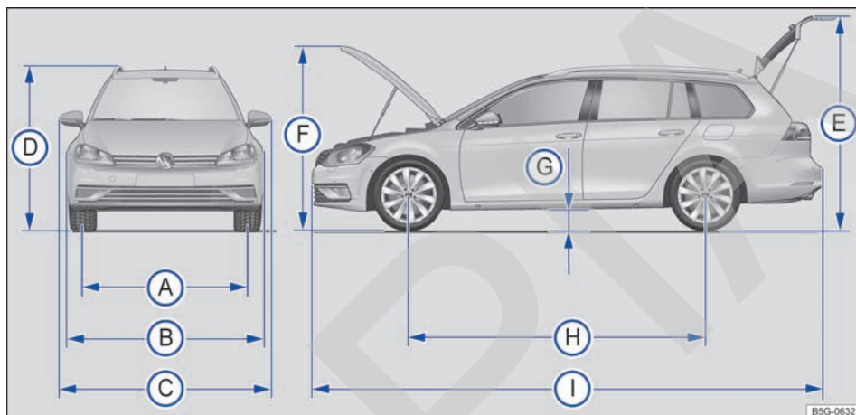
Fig. 251 Dimensiones.
