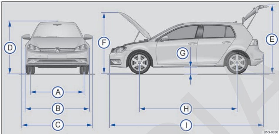
Fig. 250 Dimensiones.
