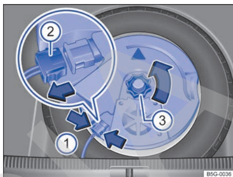
< Fig. 155 En el maletero: desmontar el subwoofer (variante 1).
