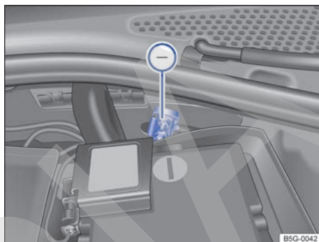
Fig. 208 En el vano motor: toma para la ayuda de arranque (terminal de masa).
