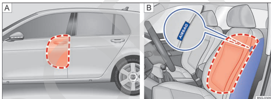
Fig. 44 [A] En el lado izquierdo del vehículo: zonas de despliegue del airbag lateral. [B] Lateral del asiento delantero: ubicación y zona de despliegue del airbag lateral.
