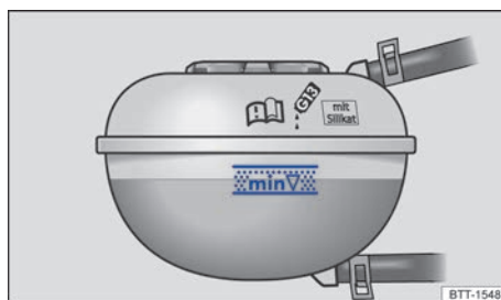
Fig. 220 En el vano motor: marcas en el depósito de expansión del líquido refrigerante del motor (representación esquemática). ▶
