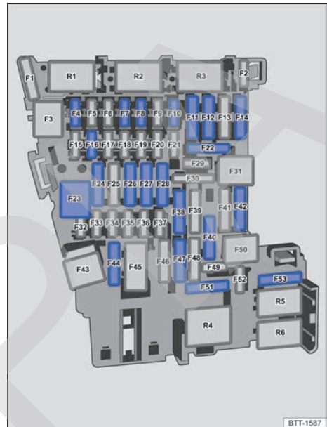
Fig. 203 En el tablero de instrumentos: asignación de fusibles.
