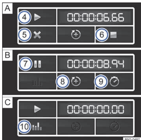
Fig. 26 Botones de función del sistema de infotainment: cronometraje en caso de una vuelta [A] detenida, [B] en curso y [C] finalizada.
