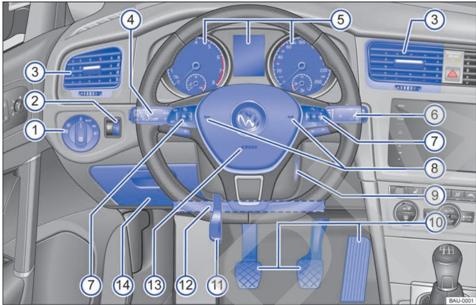
Fig. 9 Cuadro general del lado del conductor.
