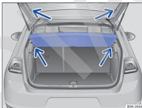
Fig. 157 En el maletero: desmontar y montar la cubierta.
