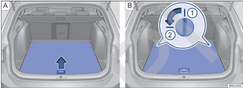
Fig. 163 En el maletero: A Levantar el piso del maletero. B Posición 1 : bloqueo del piso del maletero cerrado, posición 2 : bloqueo abierto.
