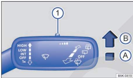
Fig. 93 En el lado derecho de la columna de dirección: palanca del limpiacristales.
