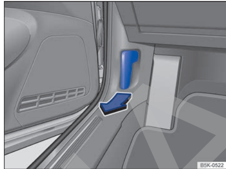
Fig. 214 En la zona reposapiés del lado del conductor: palanca de desbloqueo del capó del motor.
