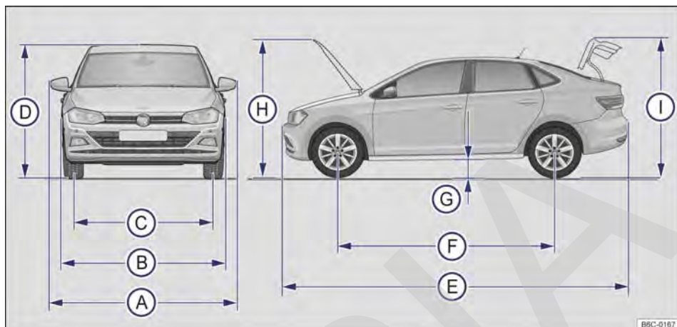
Fig. 174 Dimensiones.
