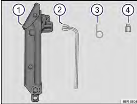
Fig. 123 Componentes de las herramientas de a bordo.
