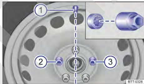
Fig. 165 Cambio de rueda: válvula del neumático ① y posición de montaje del tornillo de la rueda anti-robo ② o ③.
