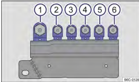
Fig. 141 En el compartimento del motor encima de la batería: disposición de los fusibles.
