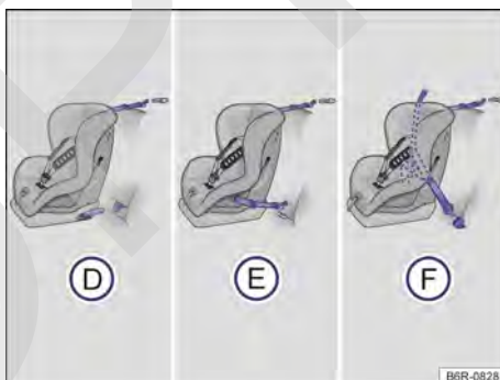
Fig. 43 En el asiento trasero: las figuras (D) y (E) muestran el principio de fijación del sistema de retención infantil en los ojales de retención inferiores y con el cinturón de fijación superior. La figura (F) muestra la fijación del sistema de retención para niños con el cinturón de seguridad del vehículo y con el cinturón de fijación superior.
